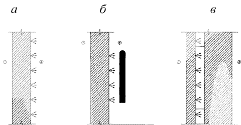
Рисунок 6.1 – Схемы эффективного размещения отрагательной теплоизоляции из алюминиевой фольги на поверхности наружной стены отапливаемого здания: на внутренней поверхности наружной стены (а); на радиаторном участке наружной стены (б); на одной из поверхностей замкнутой воздушной прослойки, расположенной ближе к наружной поверхности (в)
