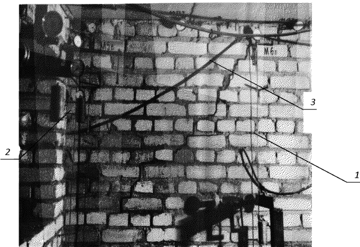
1 – внутренняя стена; 2 – наружная стена; 3 – отдельная наклонная трещина Рисунок 2 – Пример кладки с отдельными деформационными трещинами, возникшими при испытании на неравномерную осадку основания на пересечении наружной и внутренней стен
