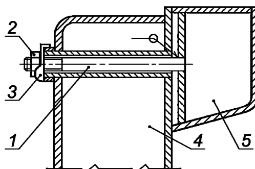
1 — шпилька; 2 — гайка; 3 — отгибная шайба; 4 — борт; 5 — вкладыш
