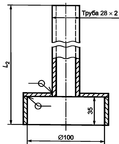
Рисунок Г.2 — Направляющая
