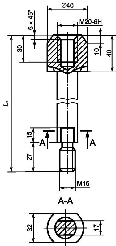
Рисунок Г.1 — Фиксатор для съемных деталей
