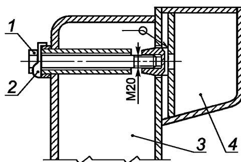
1 — болт; 2 — отгибная шайба; 3 — борт; 4 — вкладыш
