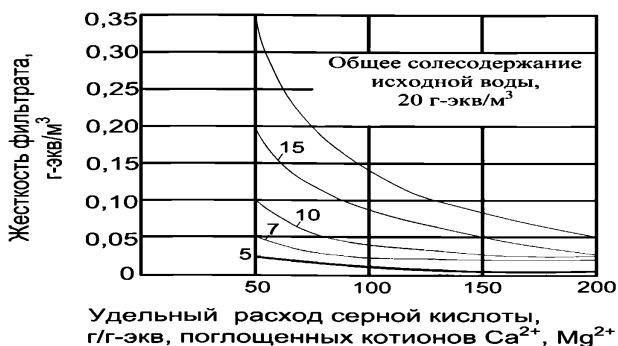
Рисунок 9.1 – График для выбора удельного расхода серной кислоты для регенерации катионита в зависимости от требуемой жесткости фильтрата
