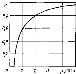
Рисунок 5.1 – Зависимость разложения \text{Na}_2\text{CO}_3 от давления в котле
