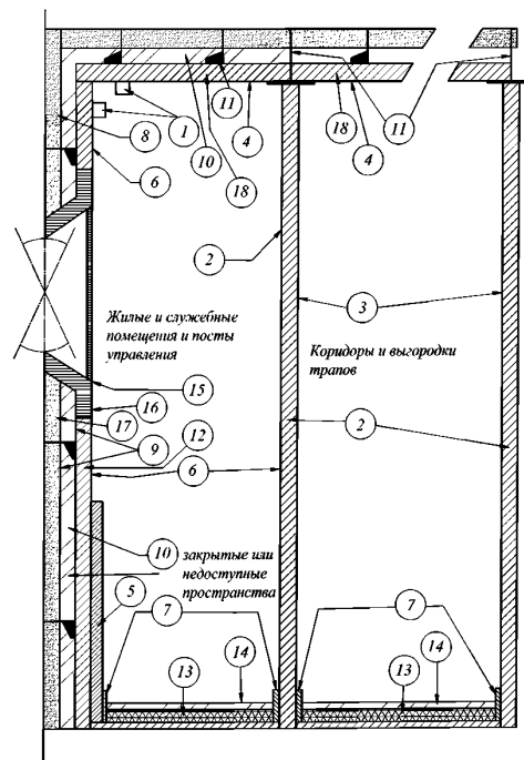
Рис. 2.3.10 Конструктивные элементы в жилых помещениях
