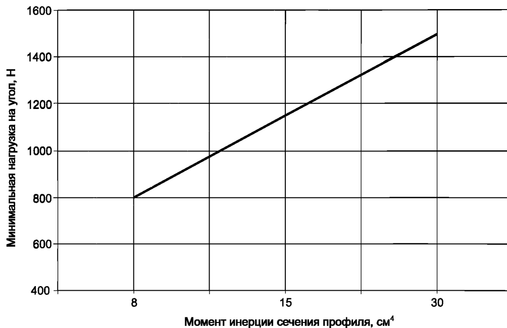
График определения нагрузки на элементы полотна
