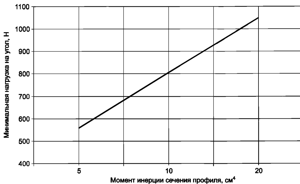
График определения нагрузки на элементы коробок
