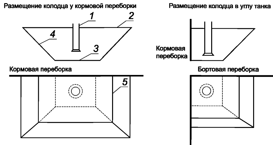
1 — труба наливная с приемным патрубком; 2 — днище грузового танка; 3 — дно колодца; 4 — наклонная стенка колодца; 5 — крышка колодца
