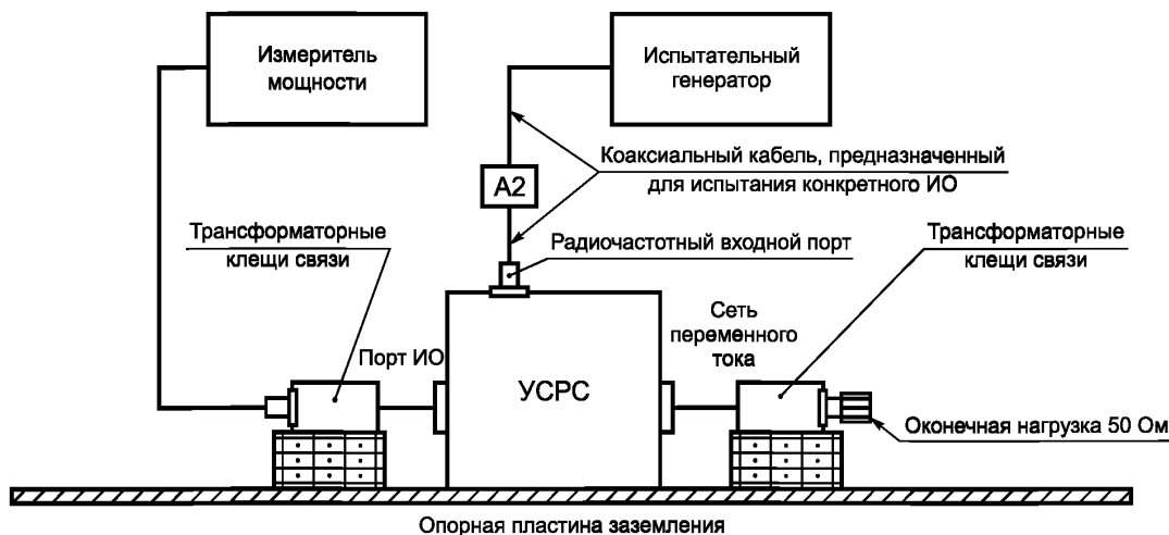
Рисунок 11 — Установка для настройки уровня сигнала
