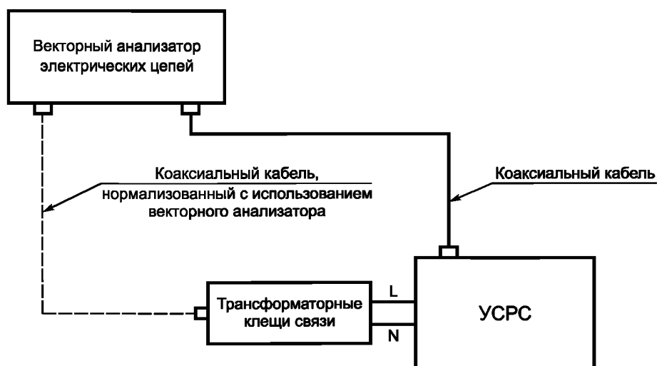
Рисунок 10 — Испытательная установка для оценки полных вносимых потерь системы ввода сигнала
