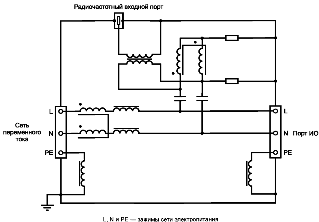
Рисунок 4 — Пример упрощенной электрической схемы УСРС
