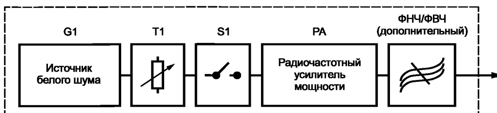
G1 — источник белого шума; T1 — переменный аттенюатор; S1 — радиочастотный переключатель; PA — радиочастотный усилитель мощности; ФНЧ/ФВЧ — фильтр низких частот и/или фильтр высоких частот (дополнительный)
