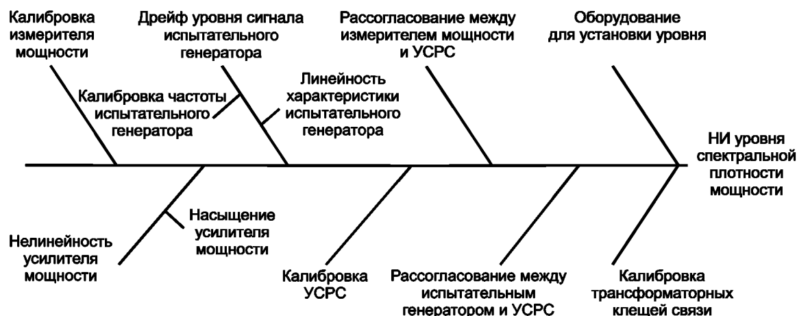
Рисунок А.1 — Примеры влияний на испытательный уровень спектральной плотности мощности при использовании УСРС
