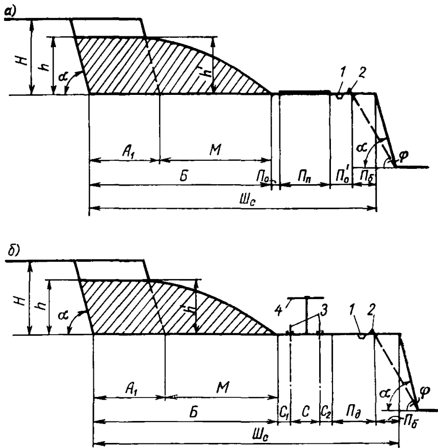
Рис. 12. Ширина рабочей площадки в скальных породах a — при автотранспорте; b — при железнодорожном транспорте; 1 — лоток (кювет); 2 — ограждение (породный вал); 3 — оси железнодорожных путей; 4 — опора контактной сети
