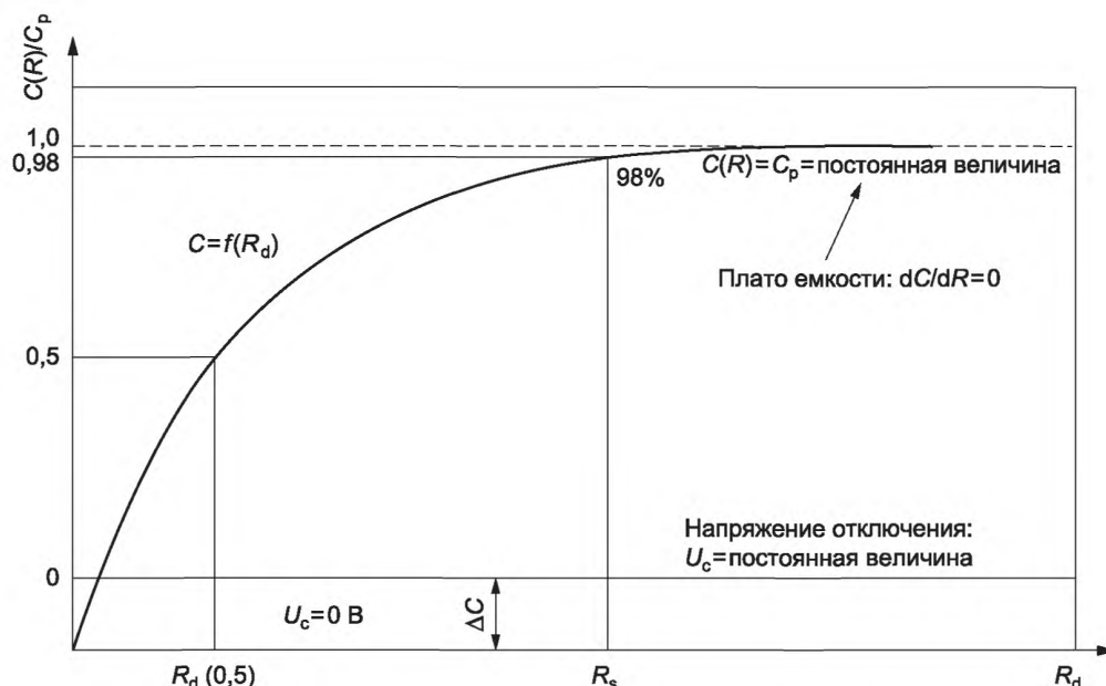
Рисунок D.1 — Нормализованная C/R диаграмма (схематично)
