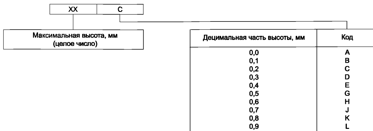
Рисунок С.7 — Код высоты, установленный в десятых долях высоты в миллиметрах
