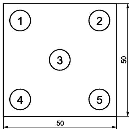
Рисунок В.2 — Схема расположения пятен при испытании методом 2 (типичная)
