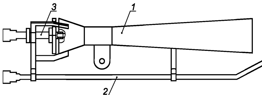
1 — диффузор, 2 — трубка поджига, 3 — сопло
