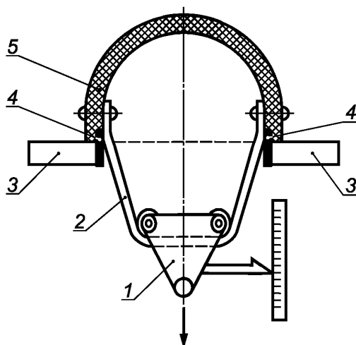
1 — приспособление; 2 — подбородочный ремень; 3 — опора; 4 — ограничитель; 5 — корпус каски
