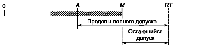
Рисунок 6 — Принцип измерения декодируемости
