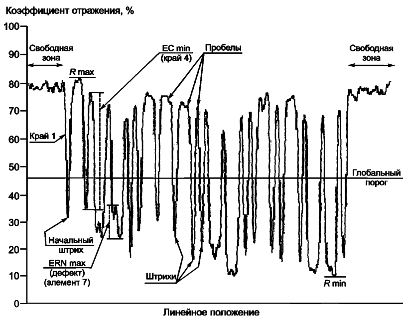
Рисунок 4 — Характерные параметры профиля отражения при сканировании
