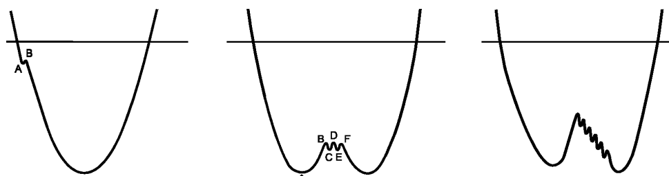
Рисунок 5 — Примеры, иллюстрирующие расчет значения ERN
