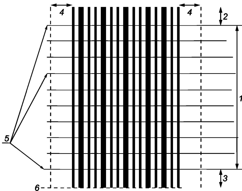
Рисунок 1 — Рекомендуемая общая оптическая схема
