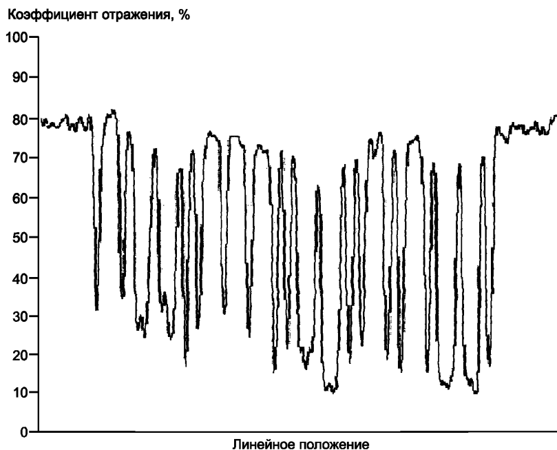
Рисунок 3 — Профиль отражения при сканировании
