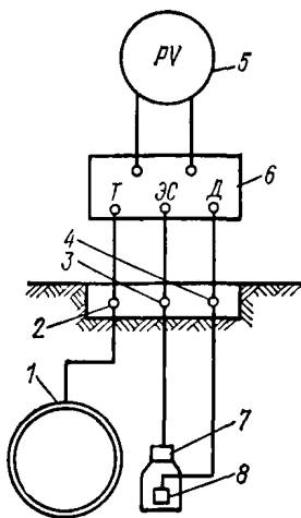
Рис. 3. Схема подключения приборов к стационарному КИП.
