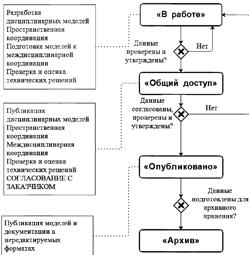
Рисунок 5 – Структура СОД
