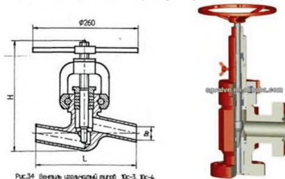
Рис.34 Игольчатый клапан КС-3, КС-4.
