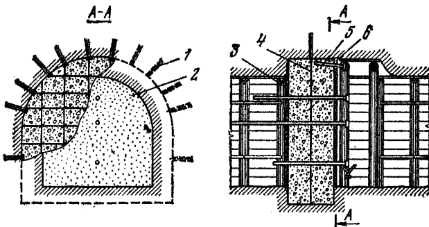
Рис. 5.13. Бетонная динамически устойчивая переемычка:
