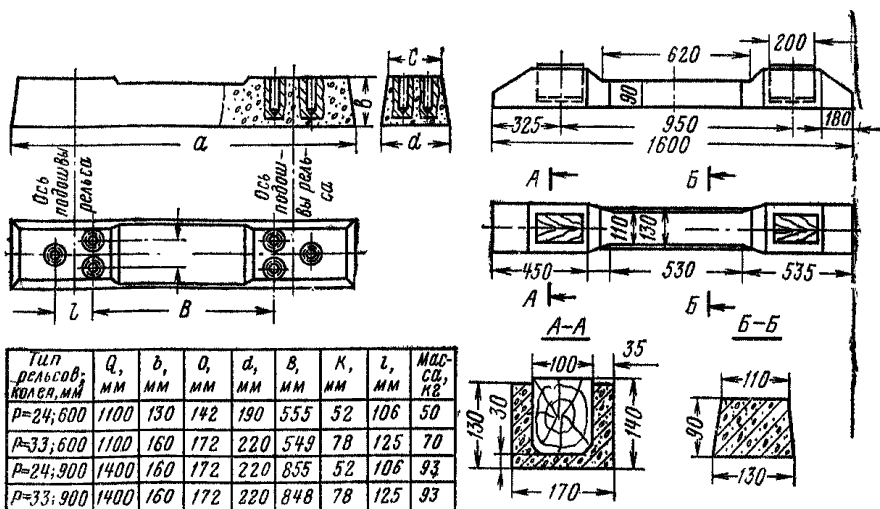
Рис. 2. Железобетонные шпалы
