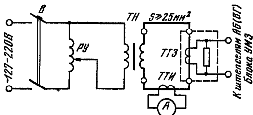
Рис. 2. Схема проверки блока защиты УМЗ:
