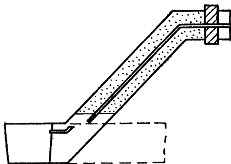
Рис. 5.2. Схема перемычки с подыливанием.
