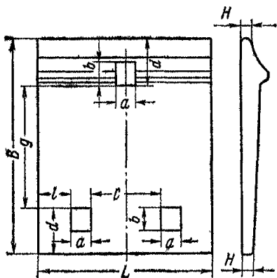
Рис. 5. Подкладка путевая одно-реборчатая
