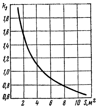
Рис. 5.3. График для определения коэффициента приведения площади перемычки
