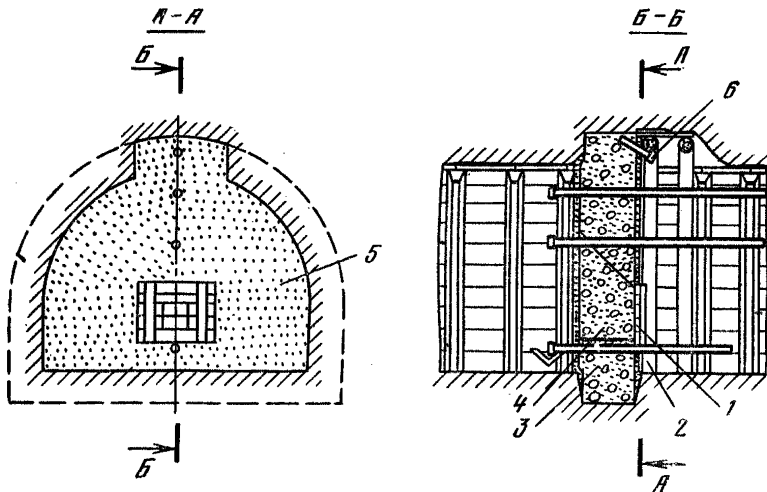
Рис. 3.18. Бетонная перемычка
