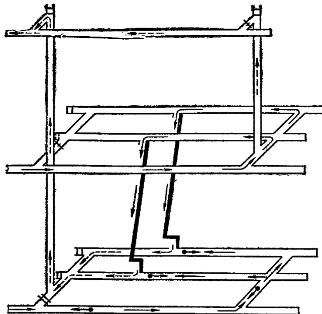
Рис. 10. Схема проветривания вентиляционного участка на крутом пласте при групповой подготовке с обособленным разбавлением и удалением вредностей и выпуском исходящей струи на вентиляционный горизонт по гезенку
