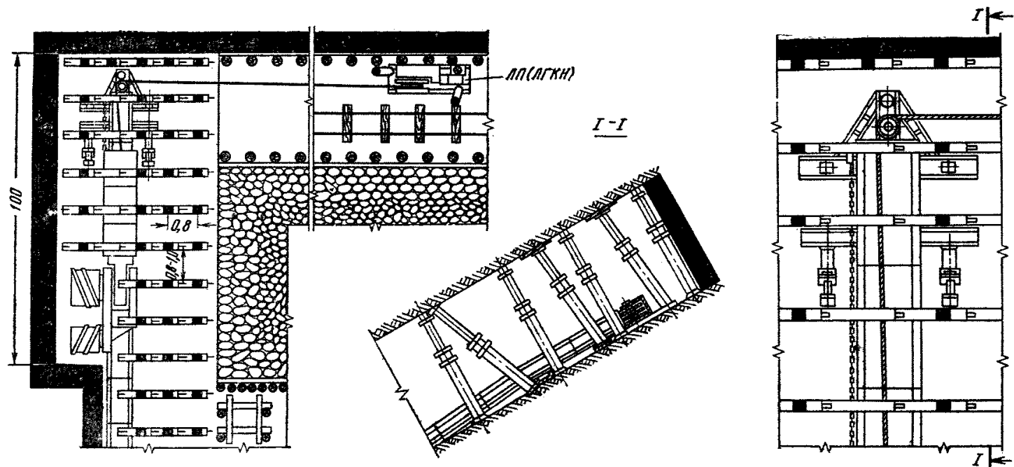
Рис. 5. Крепление тяговой цепи комбайна и обводного блока предохранительного каната на специальной раме верхнего решета
