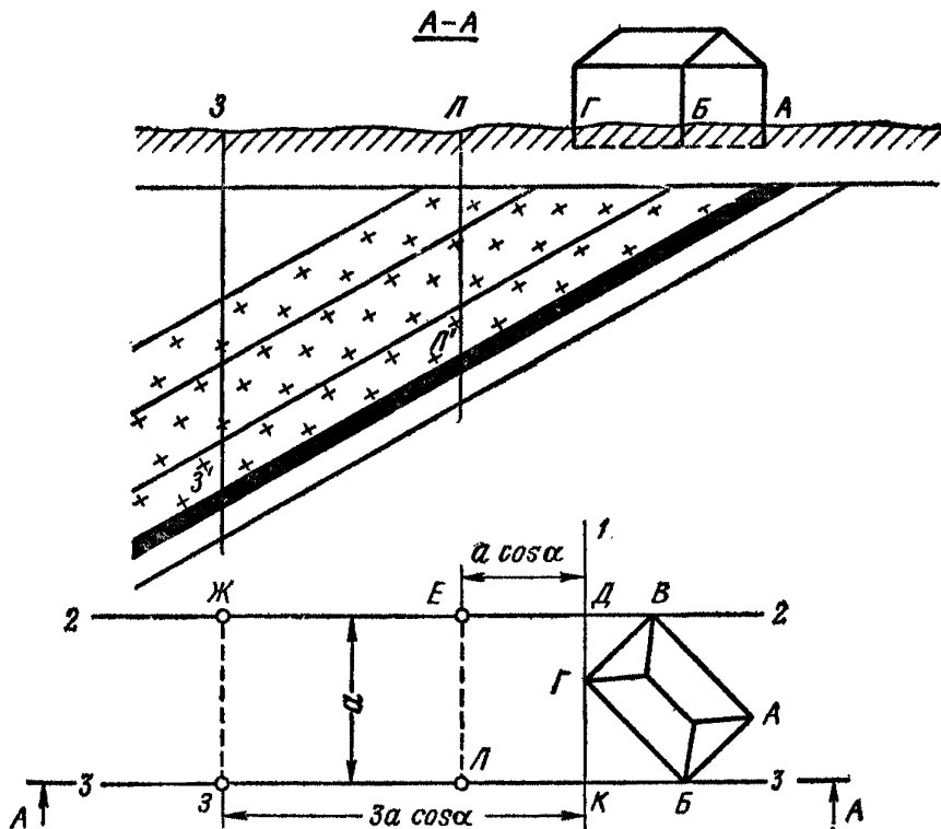
Рис. 5. Схема расположения открытых скважин
