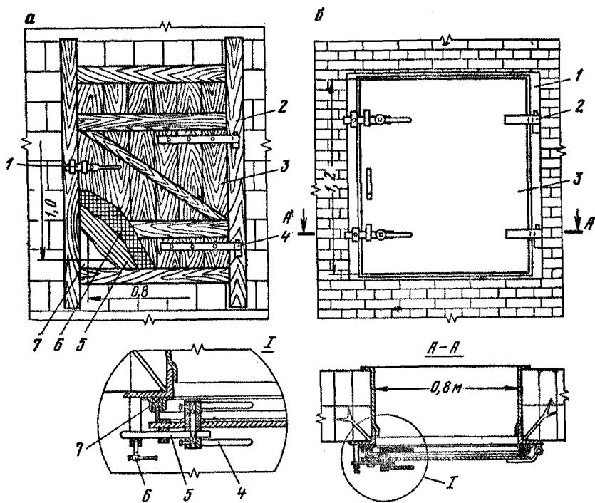
Рис. 2.5. Двери для изолирующих перегородок:
