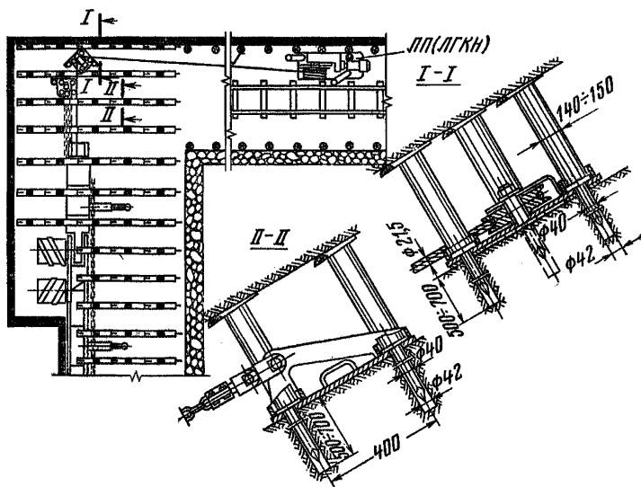
Рис. 3. Крепление тяговой цепи комбайна и обводного блока предохранительного каната на плитах, не связанных с решетчатым ставом
