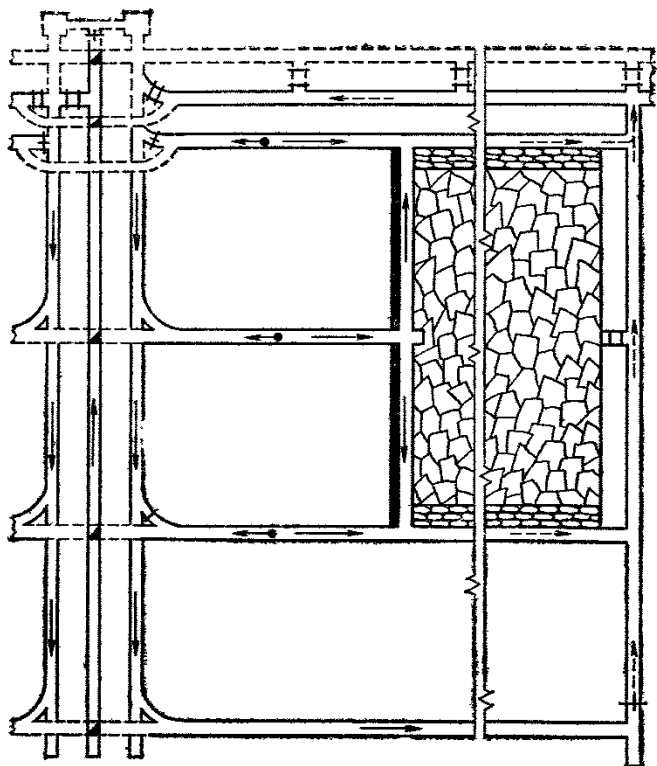
Рис. 9. Схема проветривания крыла уклонной панели с обособленным разбавлением и удалением вредностей при отработке яруса спаренными лавами нисходящим направлением струи воздуха по одной из них и выпуском исходящей струи в фланговую выработку
