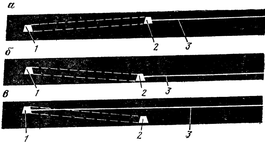
Рис. 2.22. Схема расположения дегазационных скважин при подготовке мощного пологого пласта с бурением скважин из:
