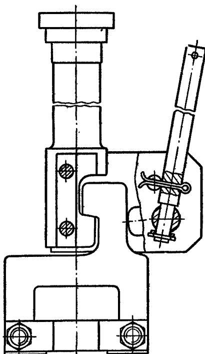
Рис. 4. Разъединительное приспособление
