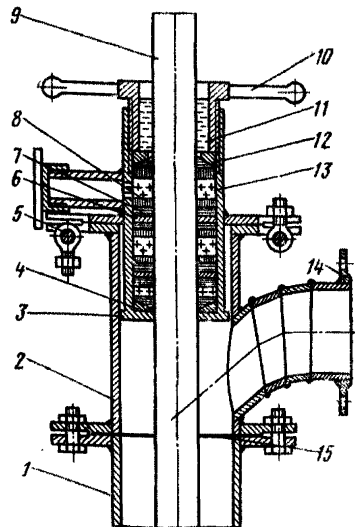
Рис. 7.1. Герметизатор
