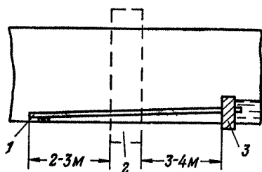
Рис. 3.11. Водоудерживающий порог: 1 — труба; 2 — перемычка; 3 — порог
