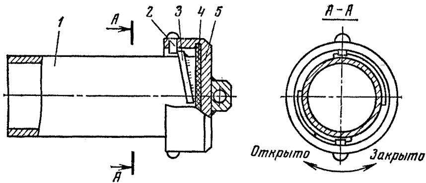
Рис. 2.4. Заглушка:
