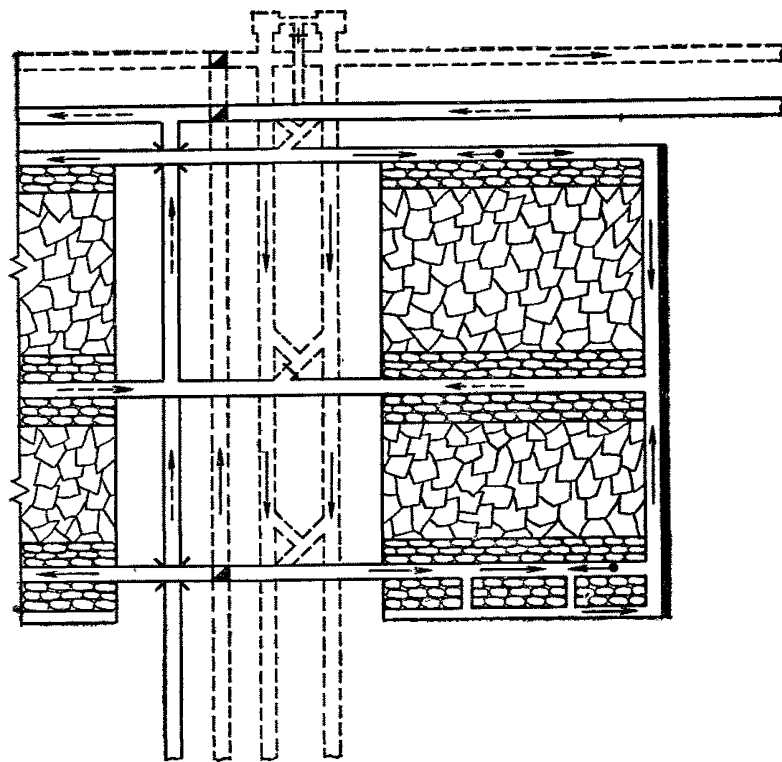
Рис. 8. Схема проветривания крыла уклонной панели с обособленным разбавлением и удалением вредностей при отработке яруса спаренными лавами и нисходящим направлением струи воздуха по одной из них
