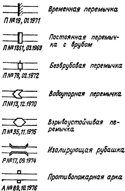
Рис. 7.1. Условные обозначения изолирующих сооружений
