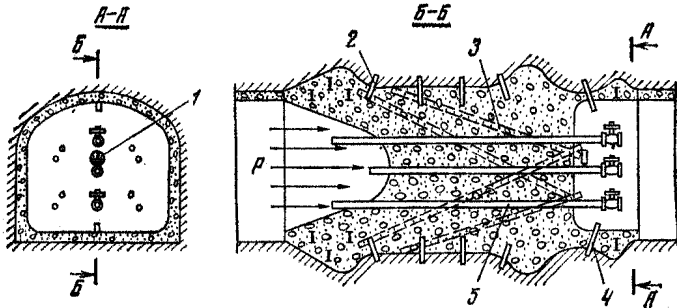
Рис. 5.10. Многослойная перемычка
