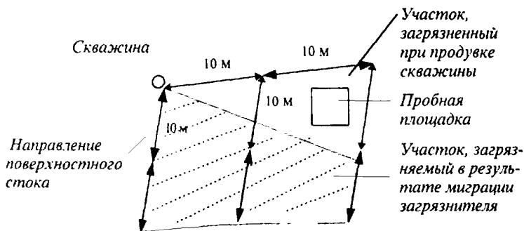
Рис. 1. Схема отбора проб вокруг эксплуатационной скважины при загрязнении нефтепродуктами
