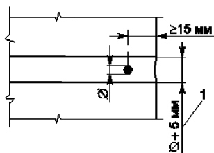
Рисунок 11.1 Защитный слой для арматуры, расположенной в горизонтальных швах
