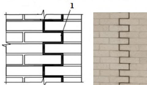
Рисунок 7.2. Устройство вертикального деформационного шва штрабой
