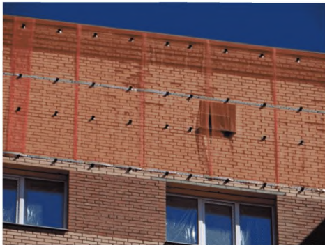
Рисунок Б.9. Защита поврежденного облицовочного каменного слоя сэндвич – панелями с низкой паропроницаемостью и высокой деформативностью при внешних температурных воздействиях
