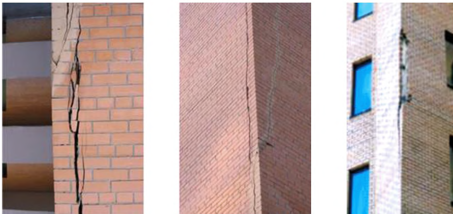
Рисунок А.1.3. Образование вертикальных и/или наклонных трещин в угловых зонах из-за отсутствия или недостаточного их армирования, отсутствия вертикальных деформационных швов
