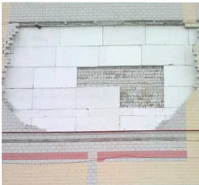
Рисунок А.1.1 Обрушение облицовочного каменного слоя из-за его недостаточного опирания, отсутствия горизонтальных деформационных швов, отсутствия либо не достаточного количества гибких связей: а – на участках с железобетонным внутренним слоем, б – на участках с каменным внутренним слоем
