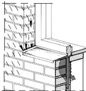
Рисунок 12.3. Зоны проникновения воды в кладку стен через не герметизированные зоны примыкания оконных блоков и водоотливов к стеновому проему
