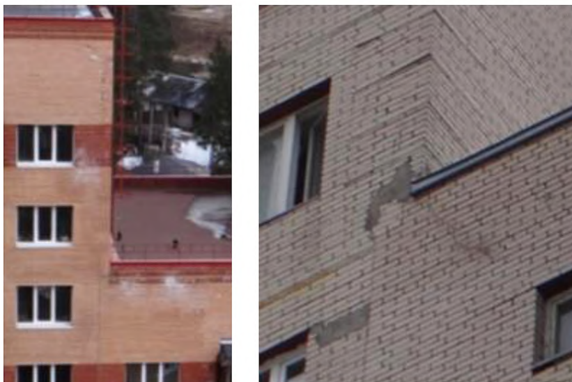
Рисунок А.1.4. Образование вертикальных и/или наклонных трещин из-за отсутствия или неправильного устройства вертикальных деформационных швов в зоне перепада высот, отсутствия или недостаточного армирования кладки в этой зоне
