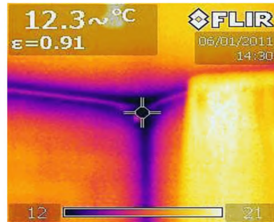
Рисунок А.1.17. Увлажнение внутри помещений из-за недостаточной теплоизоляции или протечек
