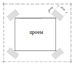
Рисунок 14.3. Дополнительное армирование штукатурного слоя в угловых зонах оконных и дверных проемов
