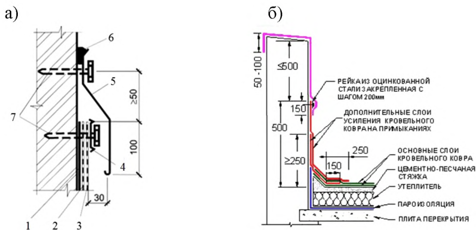
Рисунок 12.1 Устройство гидроизоляционной защиты каменного парапета
