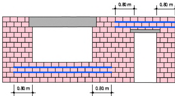
Рисунок 11.6 Горизонтальное армирование стен в зоне оконных и дверных проемов
