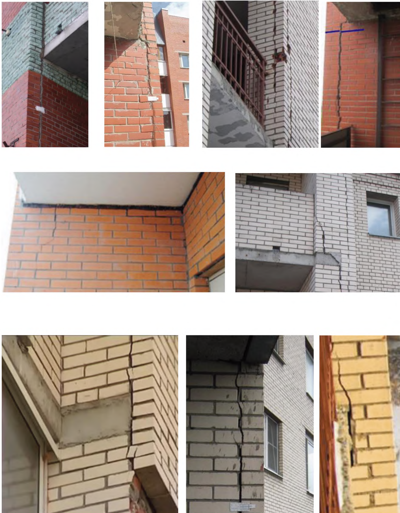
Рисунок А.1.5. Вертикальные угловые трещины в зоне выхода плит лоджий вследствие разности деформаций в перевязанном сечении кладки из-за различных условий ее опирания
