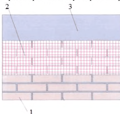
Рисунок 11.9. Фрагмент каменной стены, армируемой сетками из композитных материалов
