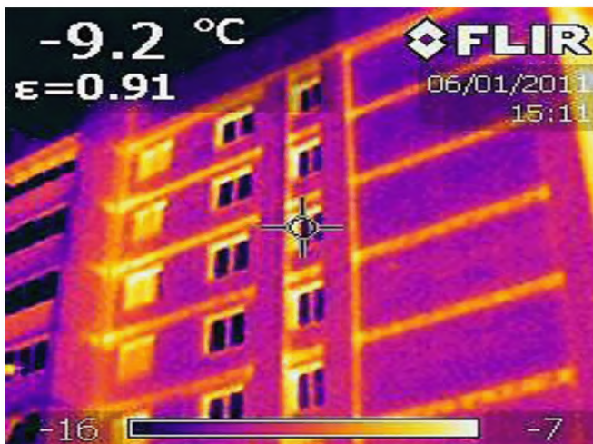
Рисунок А.1.18. Теплопотери через торцы железобетонных плит перекрытий и перемычки
