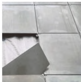
Рисунок В.2. Обрушение облицовки из керамогранита из-за слабого крепления
