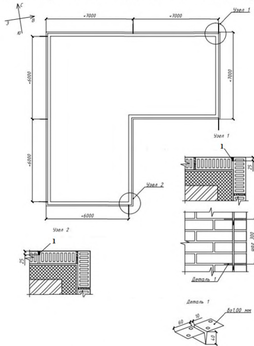
Рисунок 7.1. Расположение вертикальных деформационных швов
