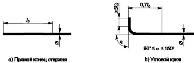
Рисунок 11.2. Анкеровка арматурных стержней в растворных швах
