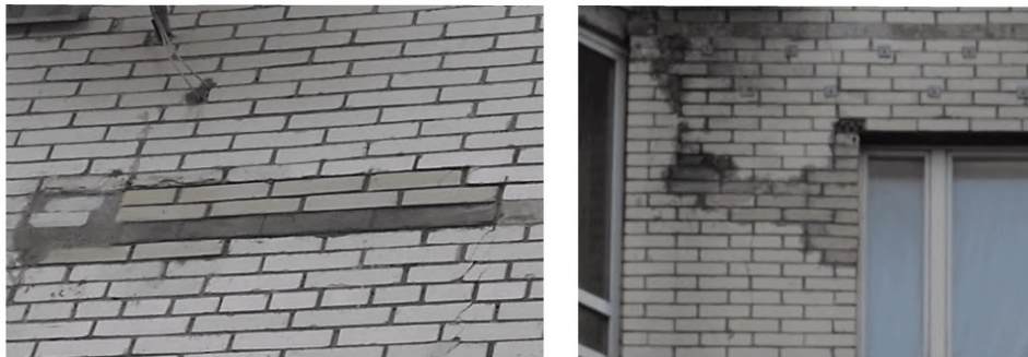
Рисунок Б.4. Ремонт облицовочного слоя с докомпановкой (заменой) разрушенных участков кладкой, отличающейся физико-механическими свойствами и цветом от основной кладки, без устранения причины разрушений или усиления фасада
