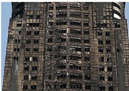
Рисунок В.11. Возгорание фасада вследствие применения горючих ветровлагозащитных мембран и композитных облицовочных кассет
