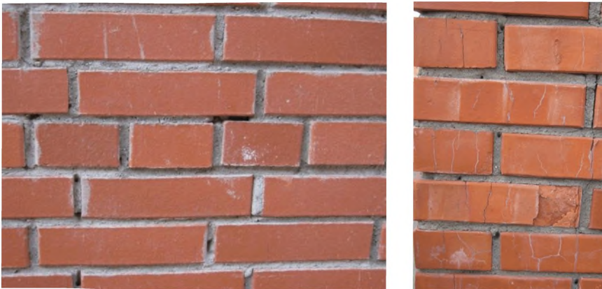
Рисунок А.2.1. Не полное заполнение горизонтальных и вертикальных растворных швов кладки (пустошовка)
