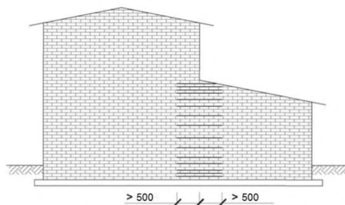
Рисунок 11.7 Армирование участка стыковки стен при перепаде высоты
