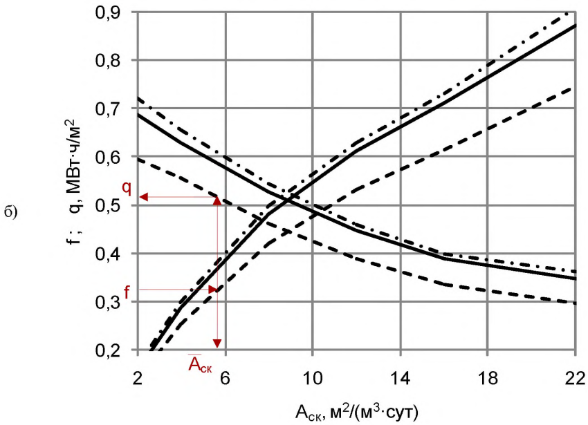
Рисунок Е.17 – Графики для определения удельной площади и годовой выработки теплоты: а) при температуре горячей воды 55 °С; б) при температуре горячей воды 30 °С.
