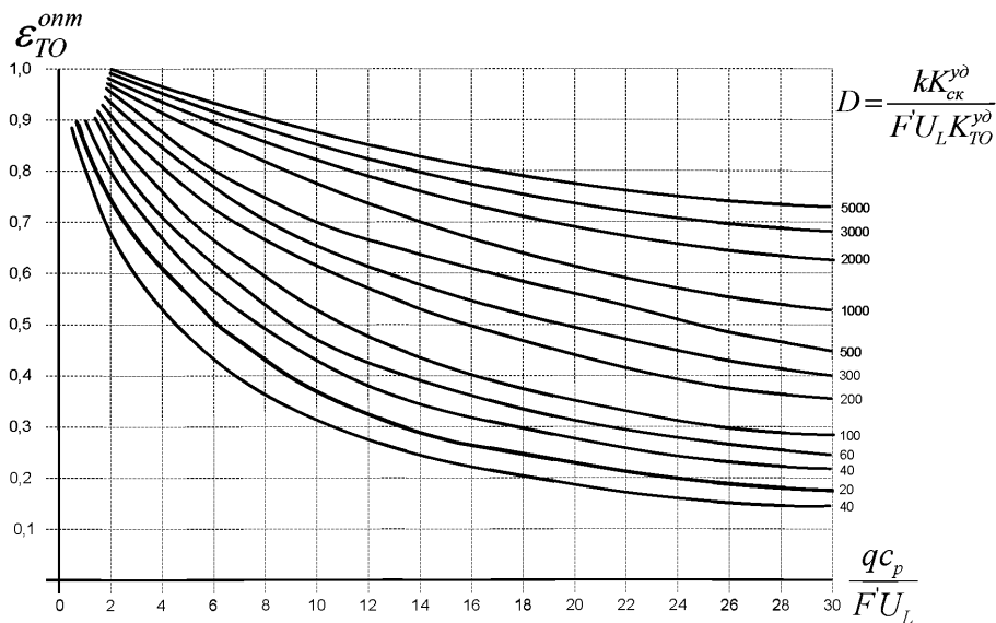
Рисунок Е.18 – График определения значения эффективности теплообменника
