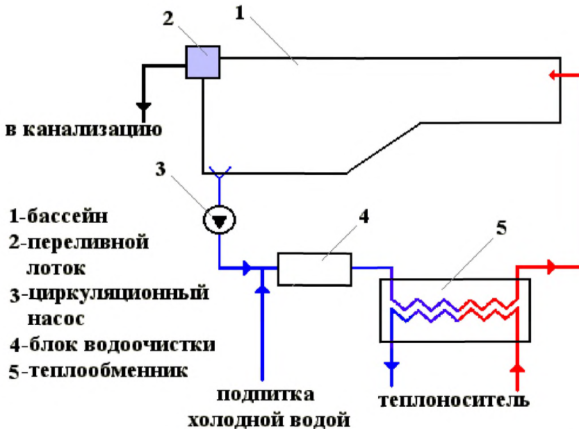
Рисунок Е.6 – Принципиальная схема оборотного водоснабжения бассейна
