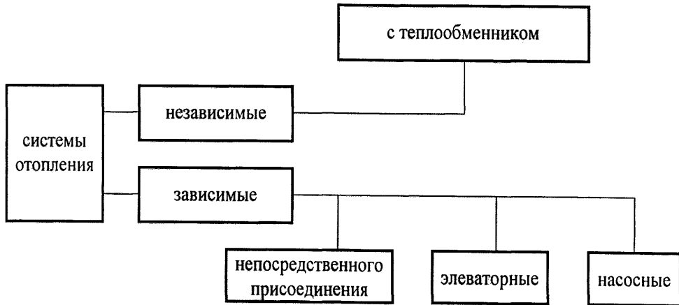
Рисунок Д.17 – Классификация систем отопления по способу присоединения к источнику теплоснабжения.
