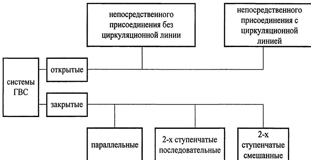
Рисунок Д.18 – Классификация систем ГВС.
