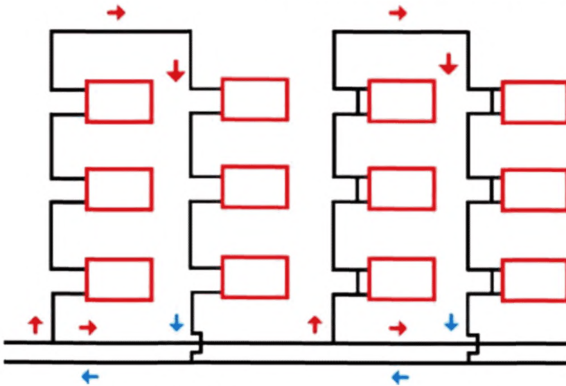
Рисунок Д.14 – Однотрубные вертикальные системы.
