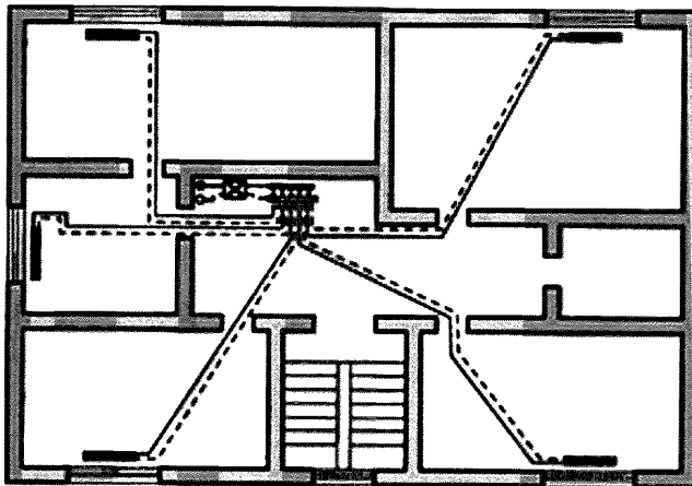
Рисунок Д.8 – Лучевая поквартирная разводка.
