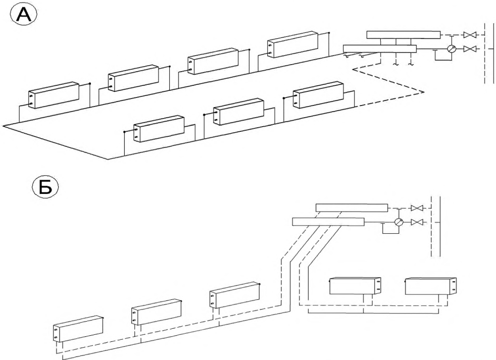
Рисунок Д.7 – Схемы разводки трубопроводов периметральных систем квартирного отопления: А – однотрубная; Б – двухтрубная.
