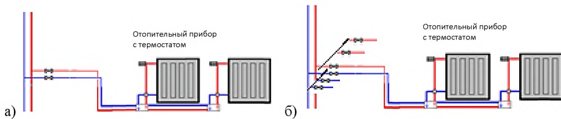
Рисунок Д.3 – Подключение внутриквартирных систем к стоякам:
