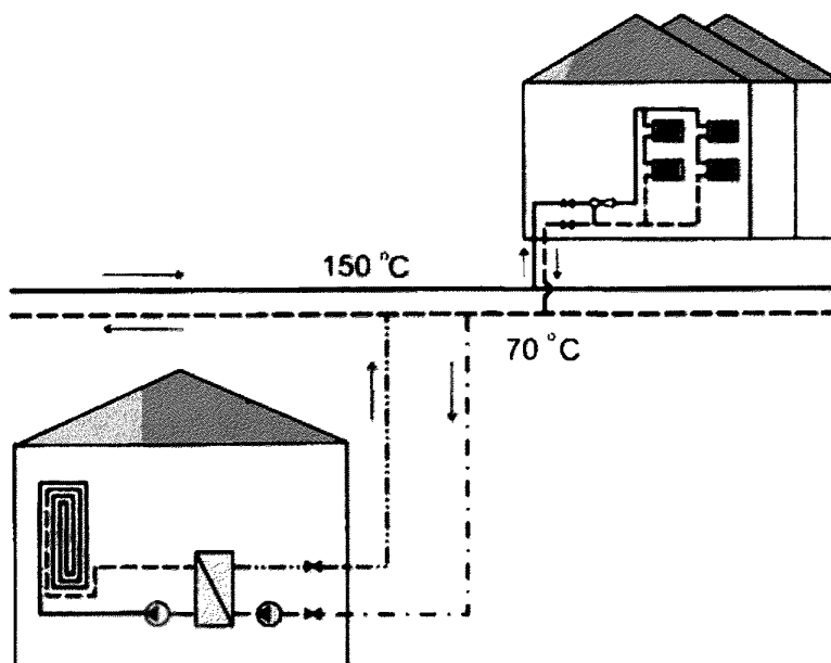
Рисунок Д.1 – Подключение здания к обратному трубопроводу тепловой сети
