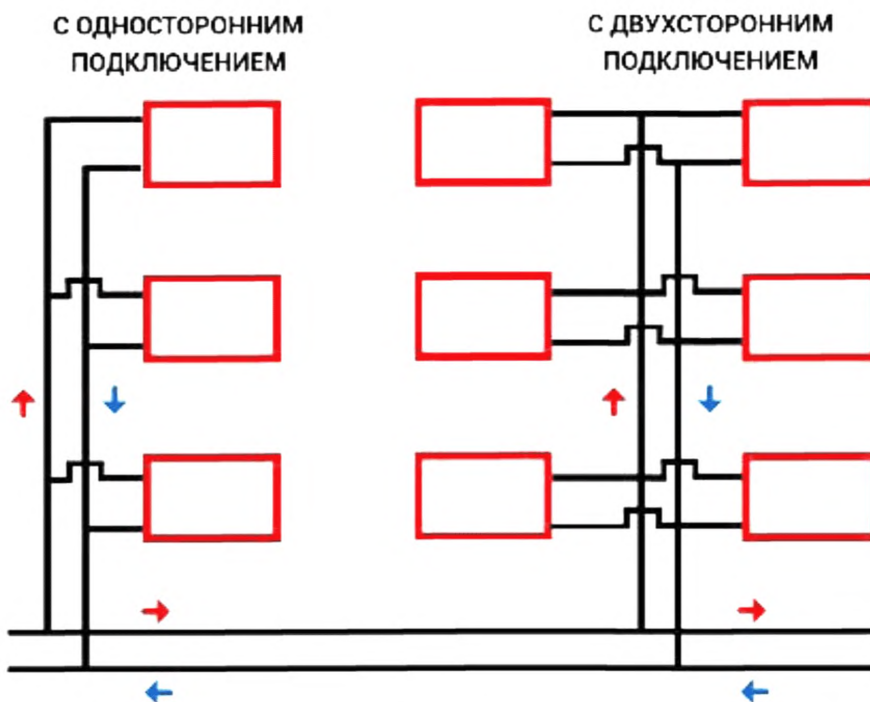
Рисунок Д.15 – Двухтрубные вертикальные системы.
