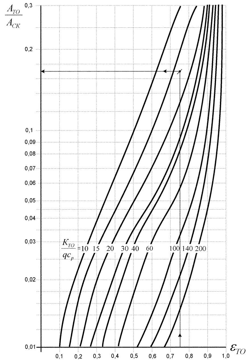
Рисунок Е.19 – График определения относительной площади теплообменника
