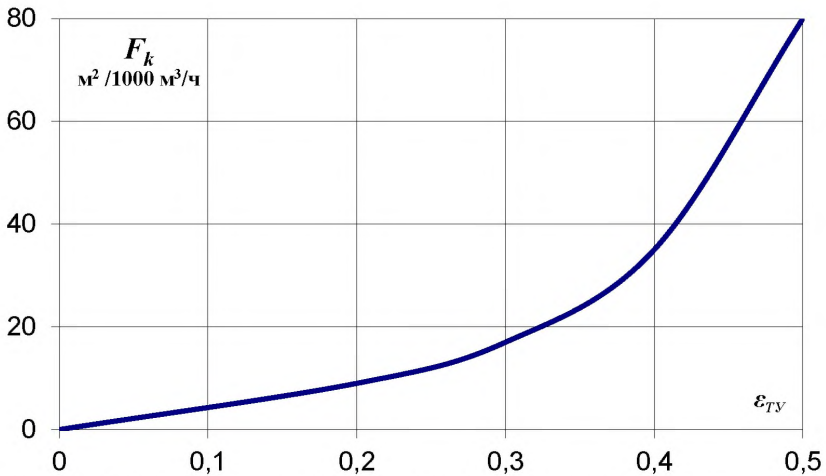
Рисунок Е.3 – Зависимость площади теплопередачи калориферов-теплоутилизаторов от степени утилизации \epsilon_{TV}
