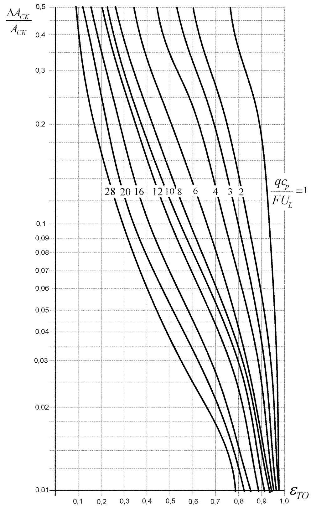
Рисунок Е.20 – Относительное увеличение площади солнечных коллекторов
