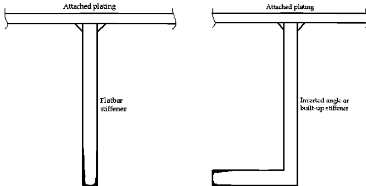
Figure 9 Edge Corrosion
