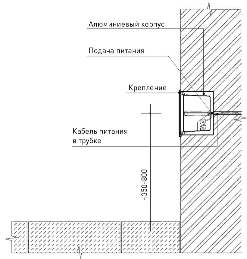
98 Схема установки встроенного светильника на стену / сечение
