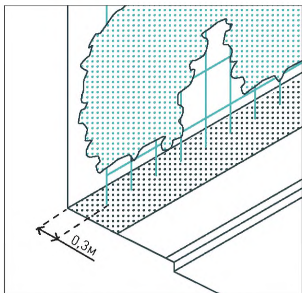
Рекомендуемое расстояние от опорных конструкций вертикального озеленения до фасадов \geq 0,3 м.
