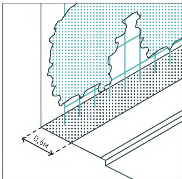
Высадка озеленения возможна в кадки или непосредственно в грунт, ширина посадочного места \geq 0,6 м.
