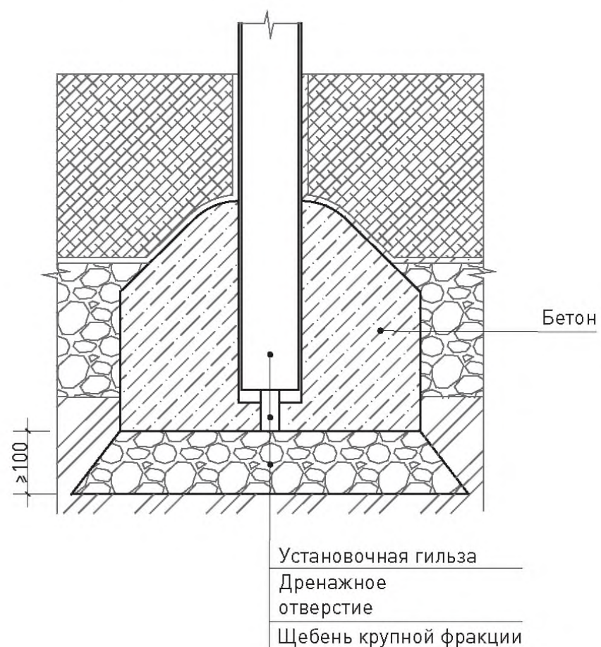
66 Схема монтажа игрового оборудования в покрытие из насыпного материала
