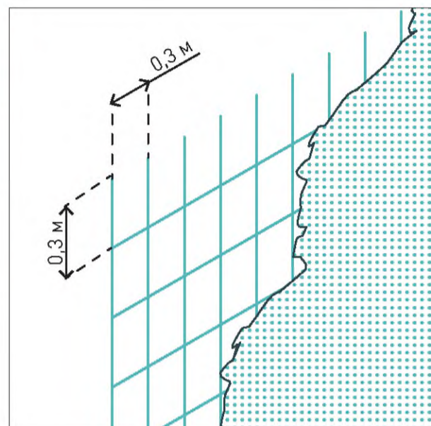
При вертикальном озеленении на шпалерах рекомендуемый шаг элементов заполнения секций — 0,3 м.
