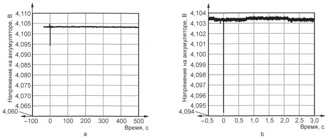
Рисунок А.31 — Напряжение в ходе испытания 14-3
