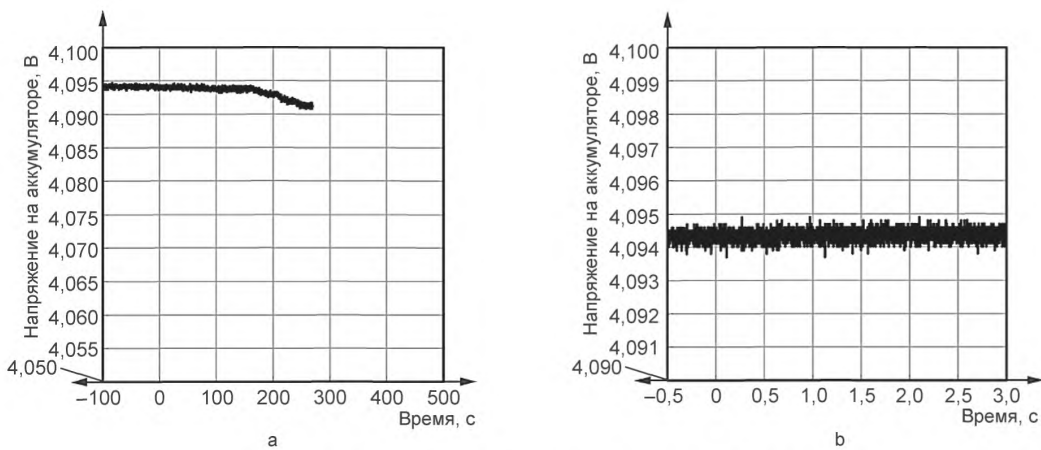
Рисунок А.32 — Напряжение в ходе испытания 14-4
