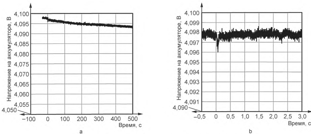
Рисунок А.33 — Напряжение в ходе испытания 14-5
