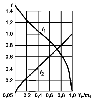
Рисунок 4.4 — График для определения коэффициентов f_1 и f_2
