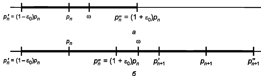
Рисунок 7.1 — Определение частот собственных колебаний
