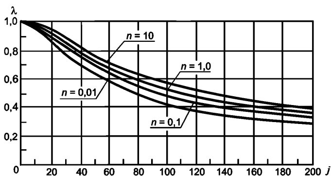
Рисунок 4.1 — График для определения коэффициента синфазности \lambda для машин и установок с асинхронными двигателями
