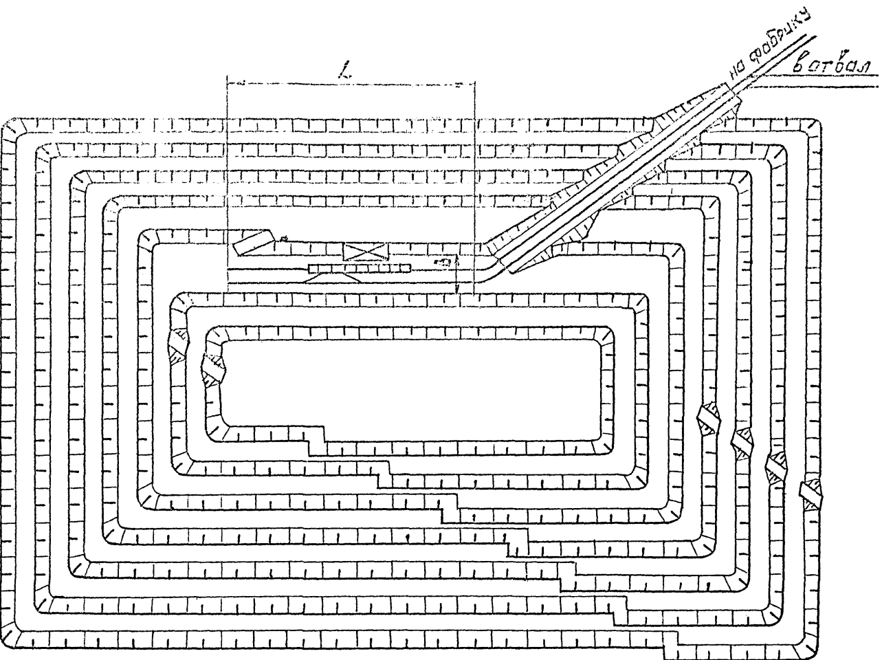
Рис. 10. Схема применения конвейерных поездов в качестве конвейерного внутрикарьерного подъёмного транспорта и на поверхности с двумя магистральными путями и челноковыми движениями по тушковой схеме с разрывной на перегрузочном пункте.
