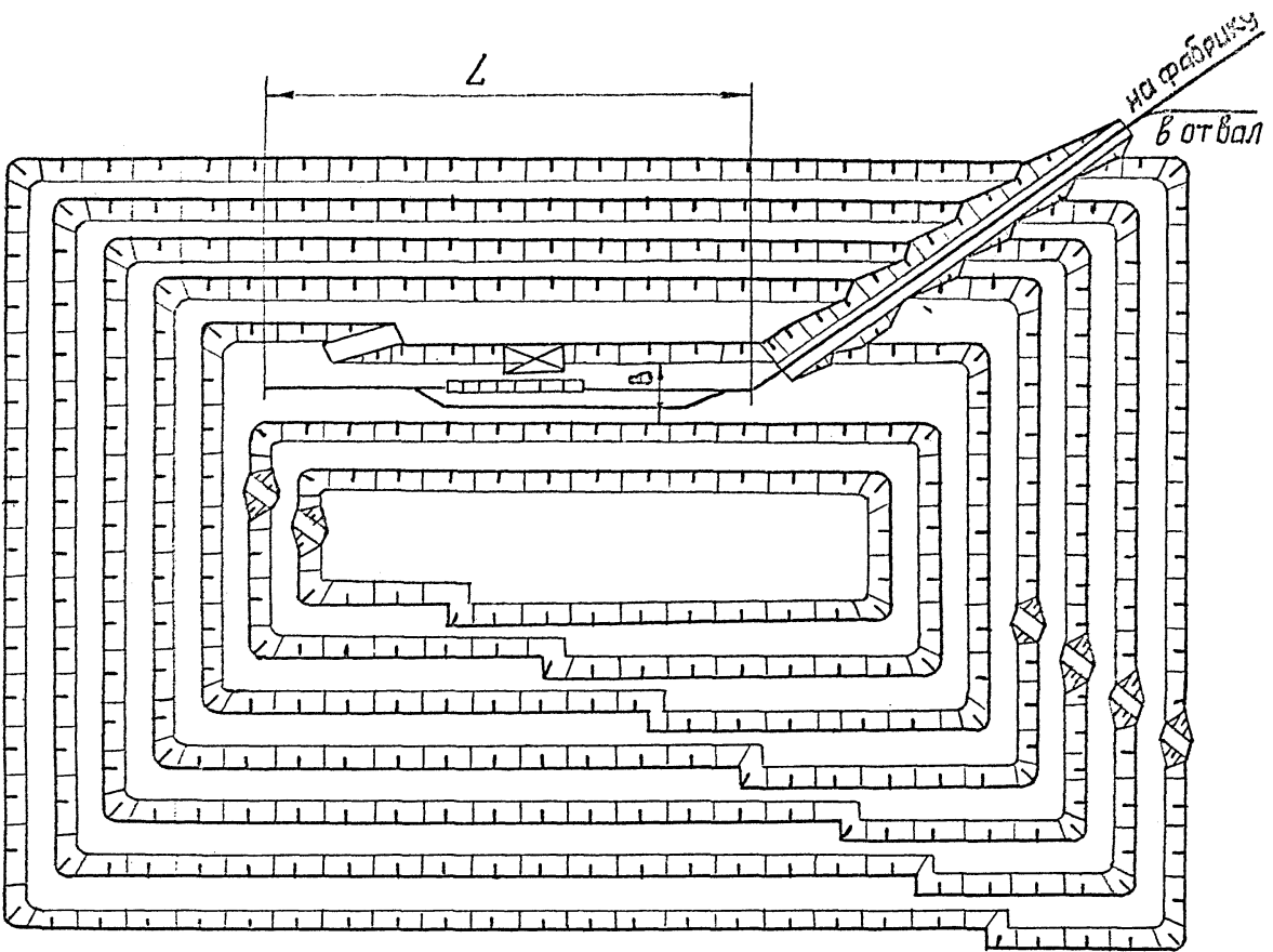
Рис. 8. Схема применения конвейерных поездов в качестве комбинированного внутрикарьерного подземного транспорта и на поверхности с челноковыми линиями по туловой схеме с разминковкой на порезгрузочном пункте.
