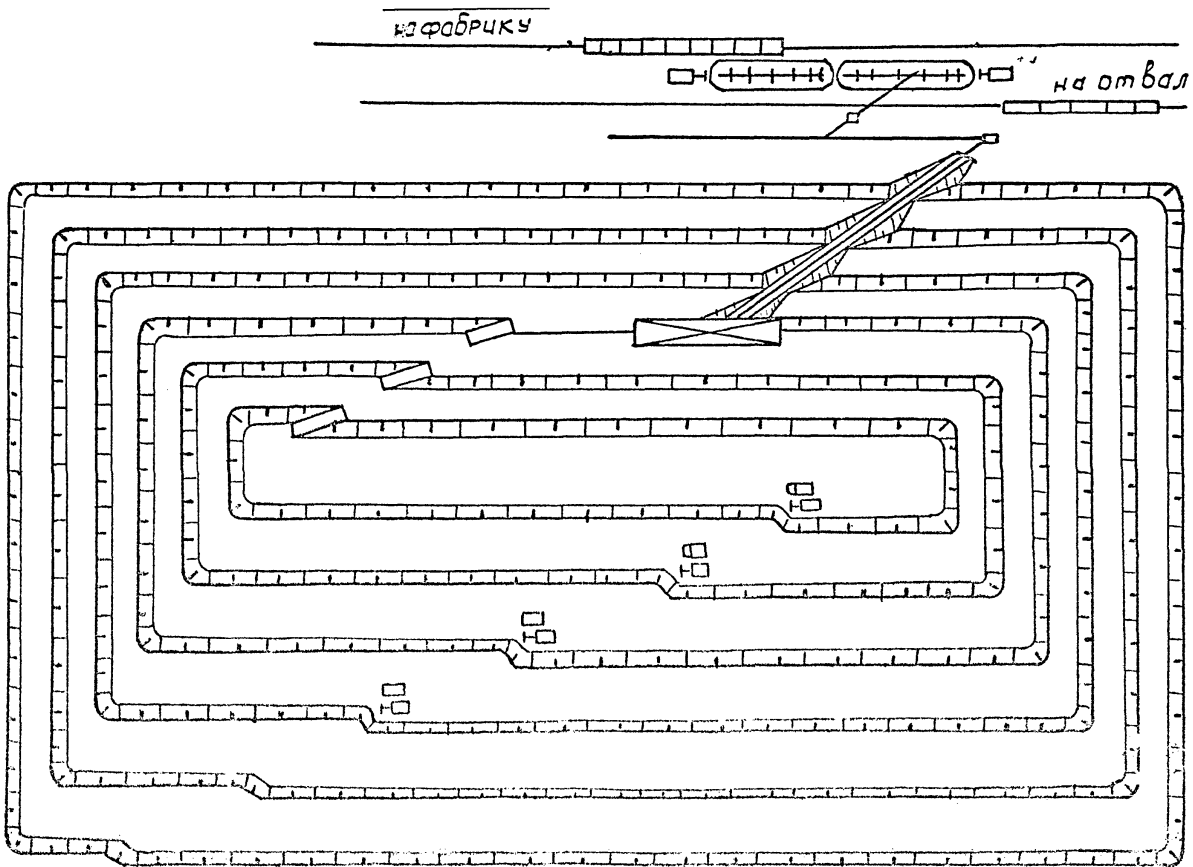
Рис. 13. Схема применения конвейерных поездов в качестве комбинированного транспортера на поверхности.
