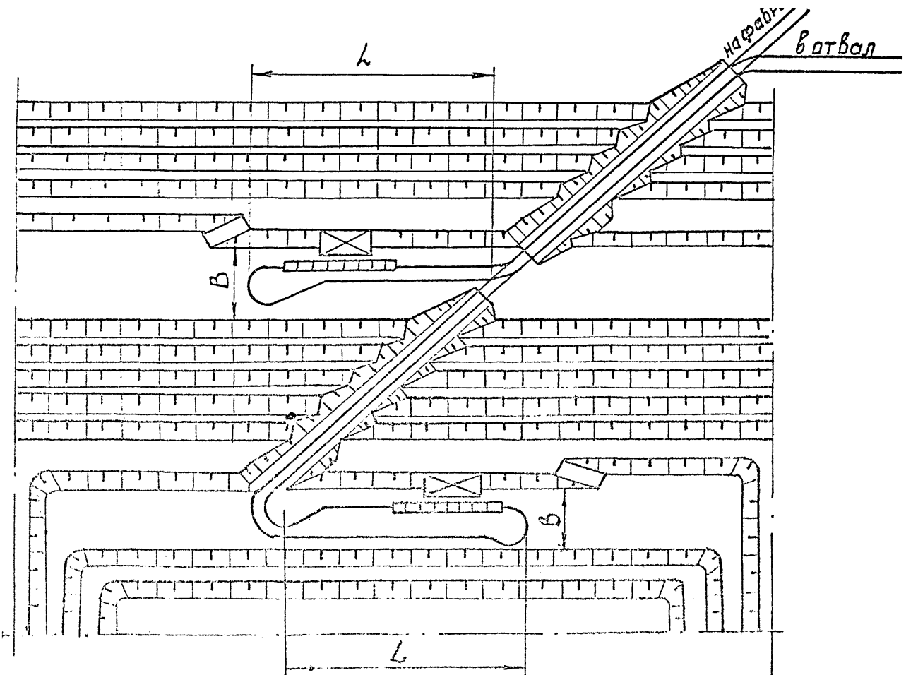
Рис. 12. Схема приления конденсера поездов в каменном комбинированного внутренкарьерного фронта и на поверхности с двумя камиральными путями и поочным движением по кольцевой схеме и дубли перегрузочными пунктами.
