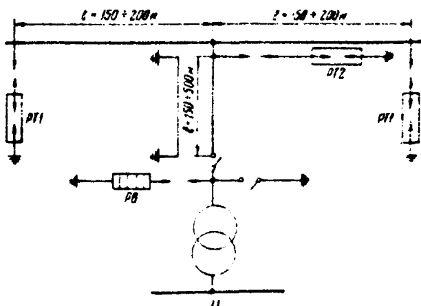
Рис.3. Схемы защиты подстанций на ответвлениях от грозных переапряжений:
