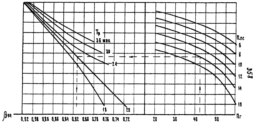
Рис. 5 Номограмма для определения коэффициента участковой скорости на двухпутных линиях, не оборудованных автобаскировкой
