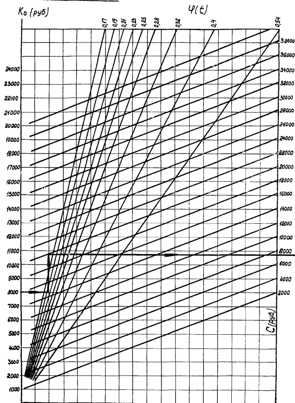
Рис. 6.1. Номограмма определения качества углеобогащающего
