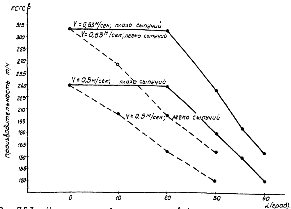
Рис. П.5.3 Номограмма зависимости производительности скребкового конвейера от ширины и скорости движения, насыпной массы материала и угла наклона конвейера
