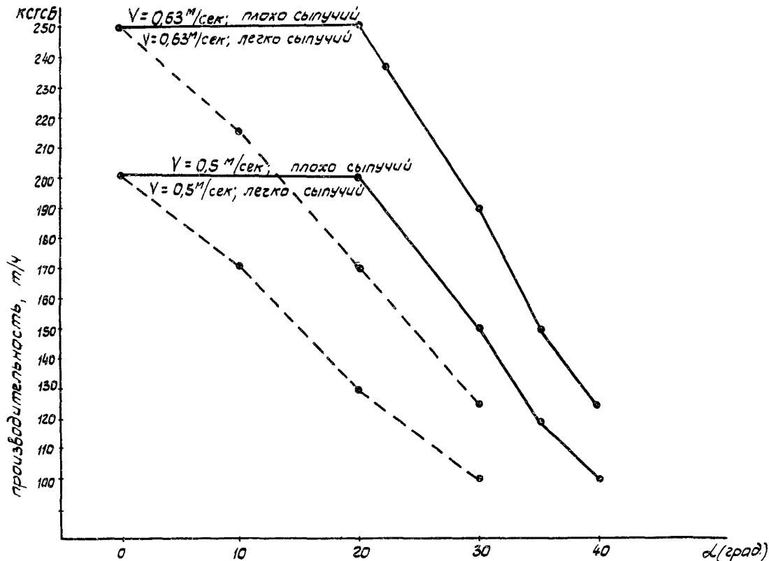
Рис. П.6.2 Номограмма зависимости производительности скребкового конвейера от ширины и скорости движения, насыпной массы материала и угла наклона конвейера — плохо сыпучий --- легко сыпучий
