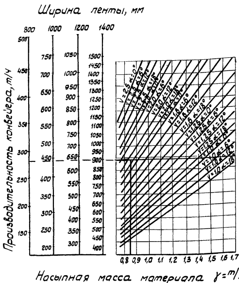
Рис. П.Б.1. Номограмма зависимости производительности ленточного конвейера от ширины и скорости движения ленты, насыпной массы материала и угла наклона конвейера
