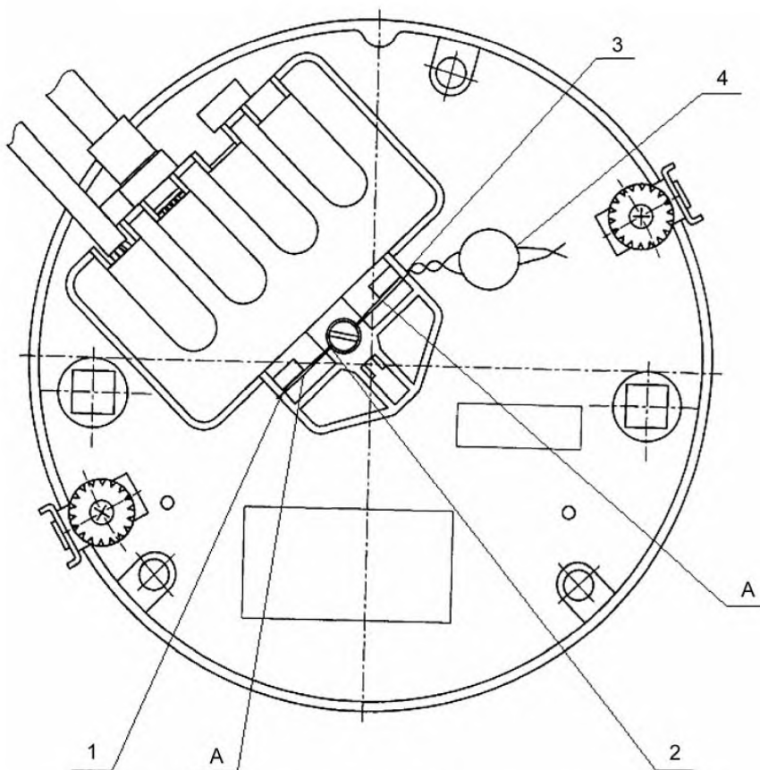
Рисунок 9 – Принципиальная схема пломбирования показывающего устройства электронного спидометра
