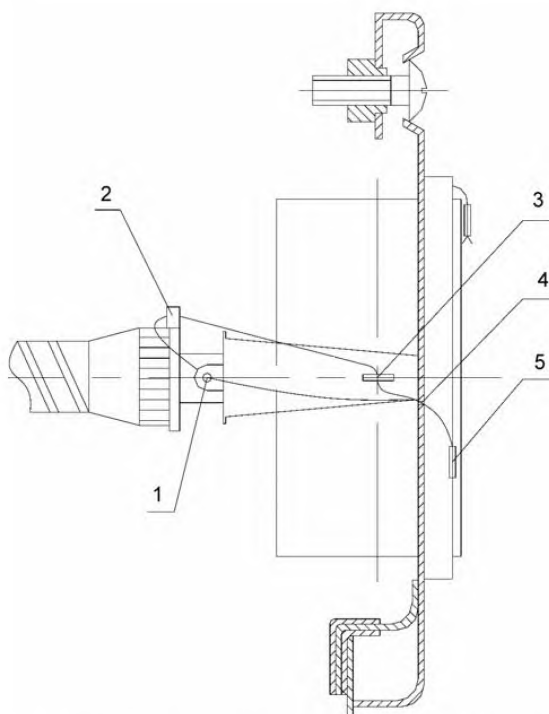
Рисунок 4 – Принципиальная схема пломбирования показывающего устройства механического спидометра
