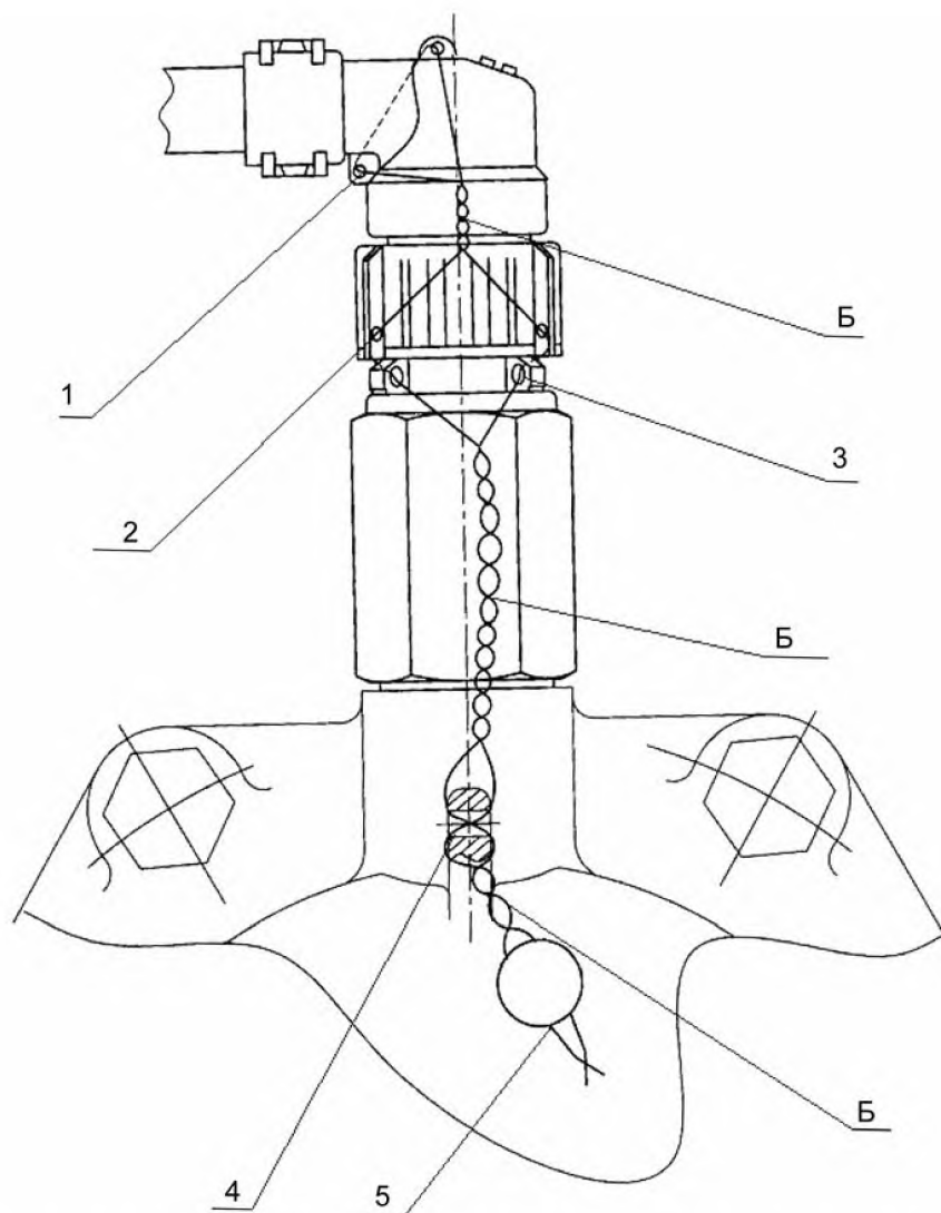
Рисунок 10 – Принципиальная схема пломбирования датчика импульсов электронного спидометра
