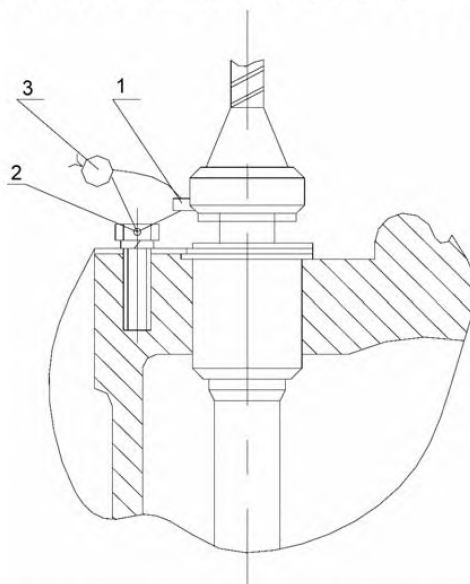
Рисунок 5 – Принципиальная схема пломбирования привода механического спидометра
