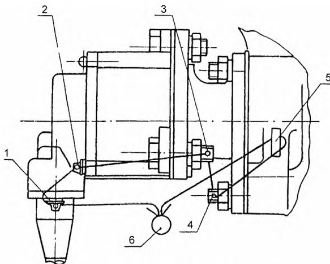
Рисунок 7 – Принципиальная схема пломбирования датчика электромеханического спидометра
