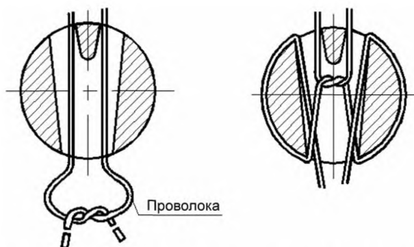
Рисунок 2 – Принципиальная схема установки свинцовой пломбы
