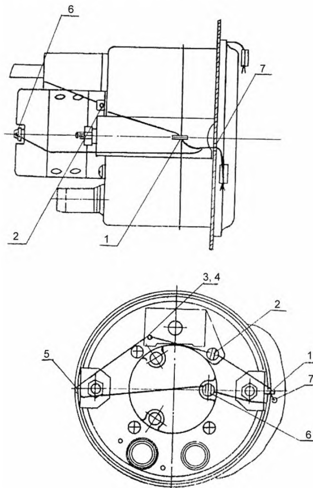
Рисунок 6 – Принципиальная схема пломбирования показывающего устройства электромеханического спидометра
