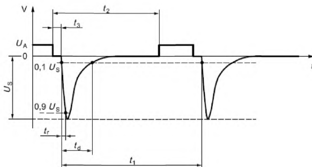
Рисунок 5 – Испытательный импульс 1
