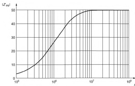
Рисунок 4 – Полное сопротивление |Z_{PB}| как функция частоты от 100 кГц до 100 МГц (AB замкнуты накоротко)
