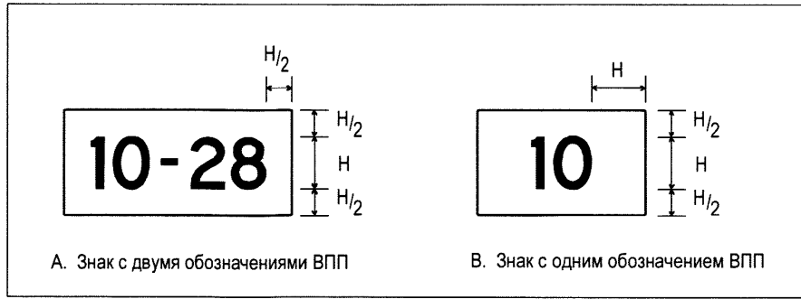
Рис. А4-4. Размеры знака
