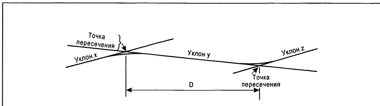
Рис. А-2. Сечение по осевой линии ВПП
