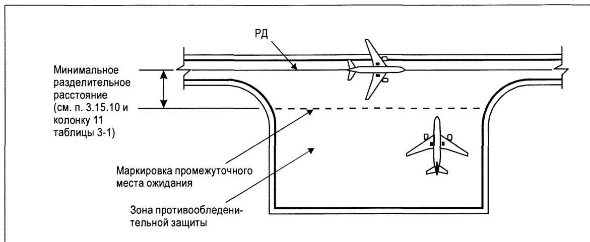
Рис. 3-4. Минимальное разделительное расстояние в зоне противообледенительной защиты
