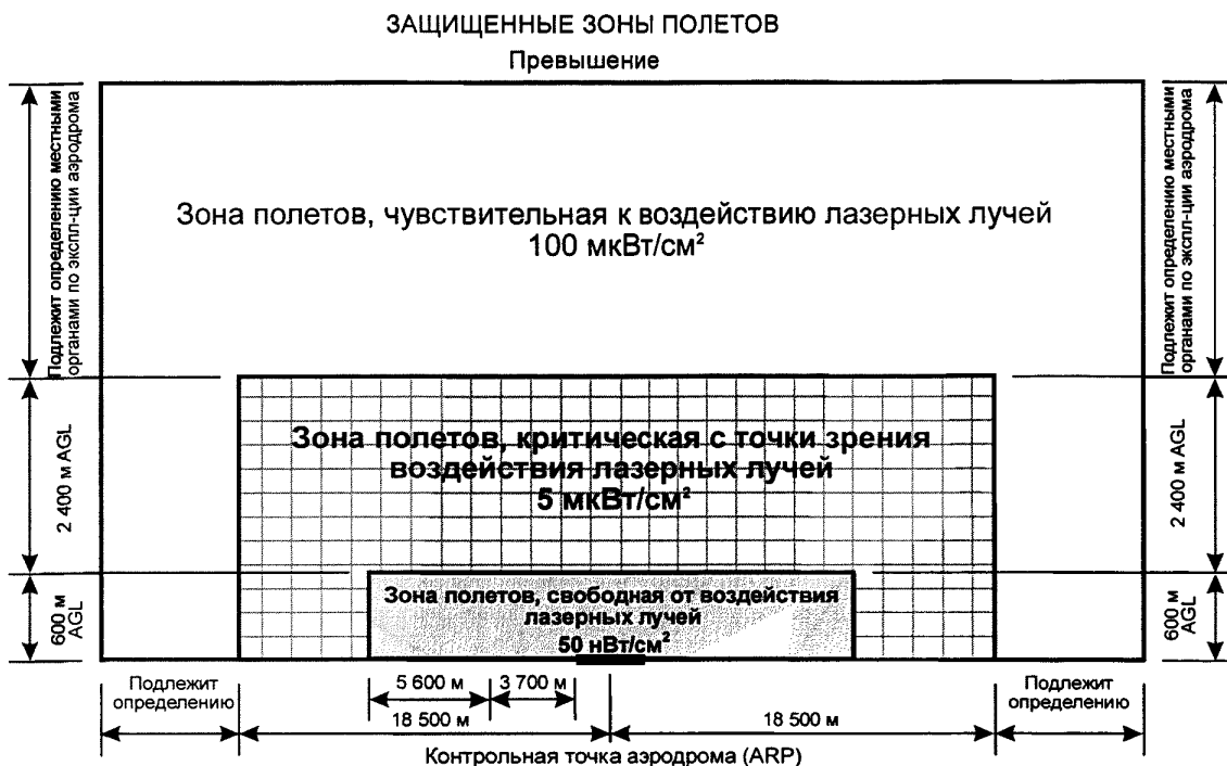
Рис. 5-13. Защищенные зоны полетов с указанием максимальных уровней излучения для видимых лазерных лучей
