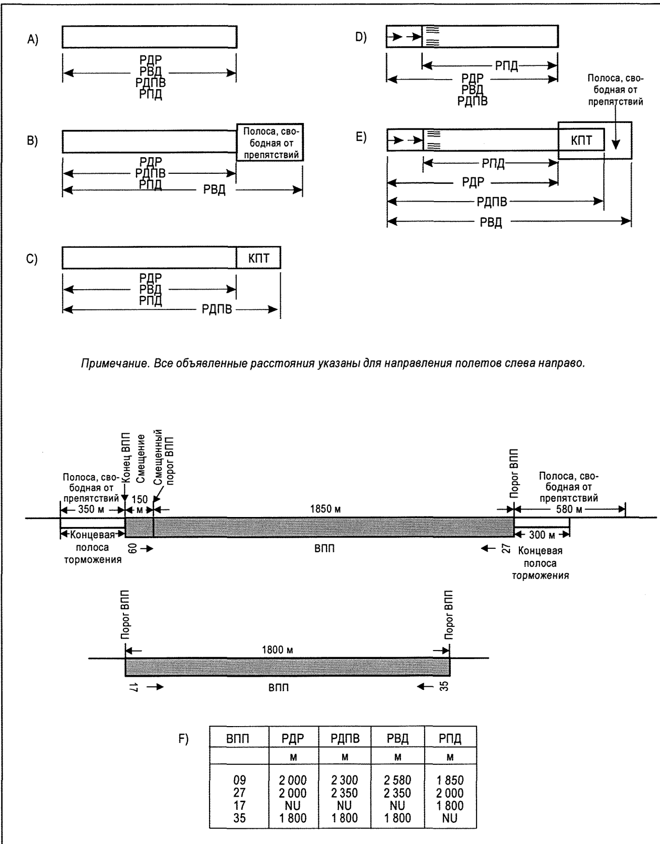
Рис. А-1. Иллюстрация объявленных дистанций
