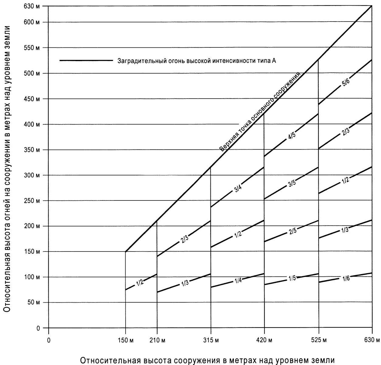
Рис. А5-6. Система светоограждения препятствий с белыми проблесковыми огнями высокой интенсивности типа А
