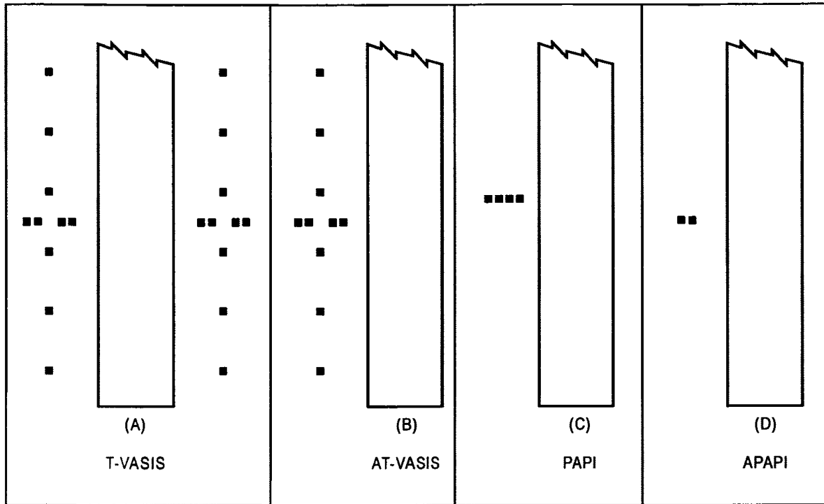
Рис. 5-16. Системы визуальной индикации глиссады
