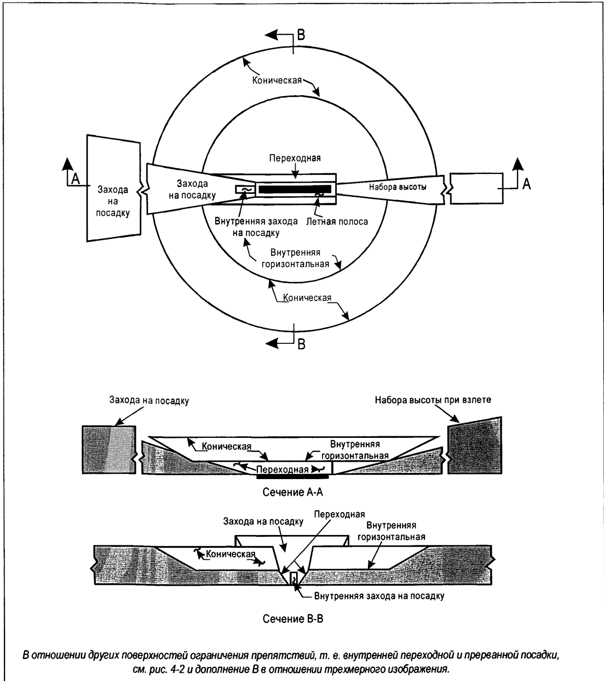
Рис. 4-1. Поверхности ограничения препятствий
