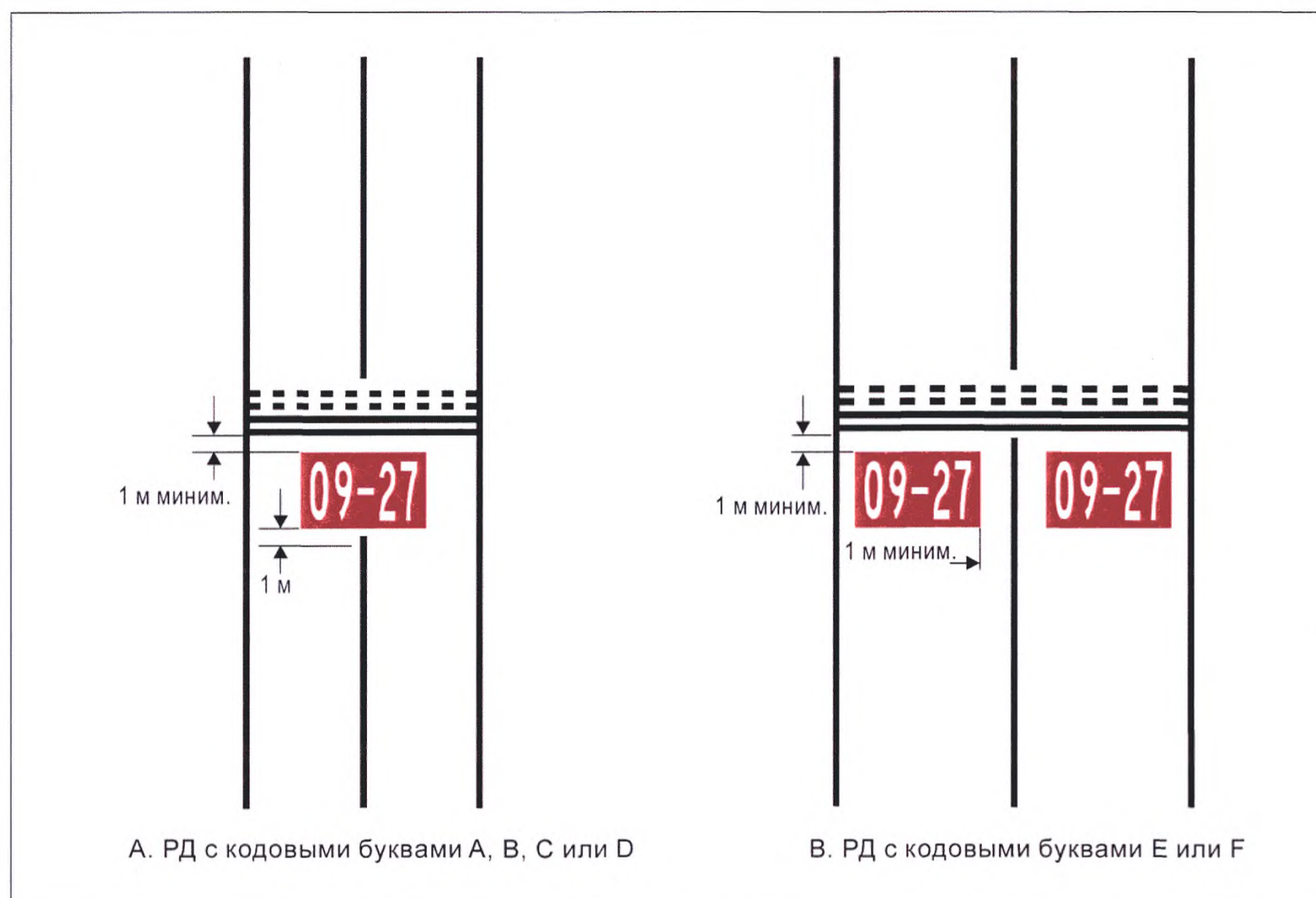
Рис. 5-10. Маркировка, содержащая обязательные для исполнения инструкции
