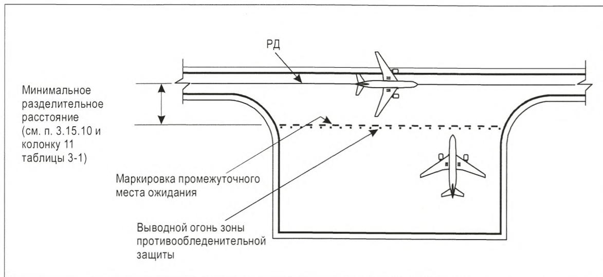
Рис. 5-28. Типичная удаленная зона противообледенительной защиты
