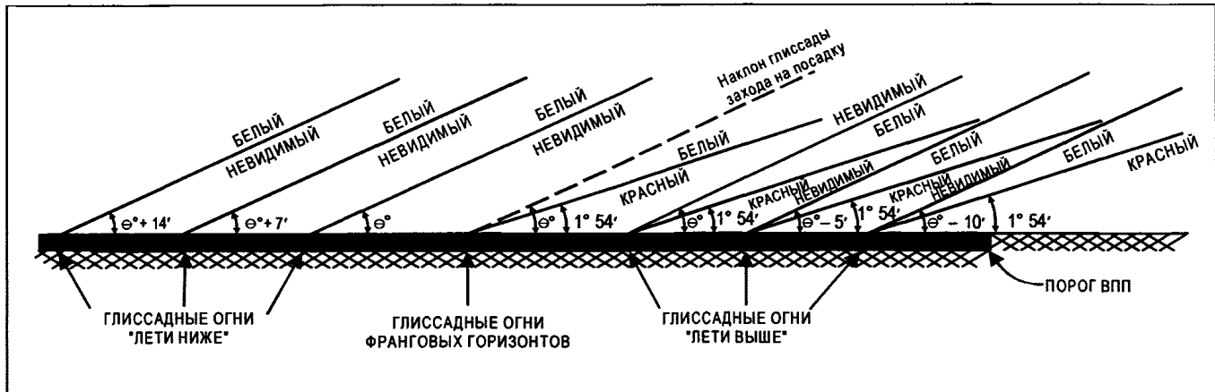
Рис. 5-18. Световые лучи и установка углов возвышения систем T-VASIS и AT-VASIS
