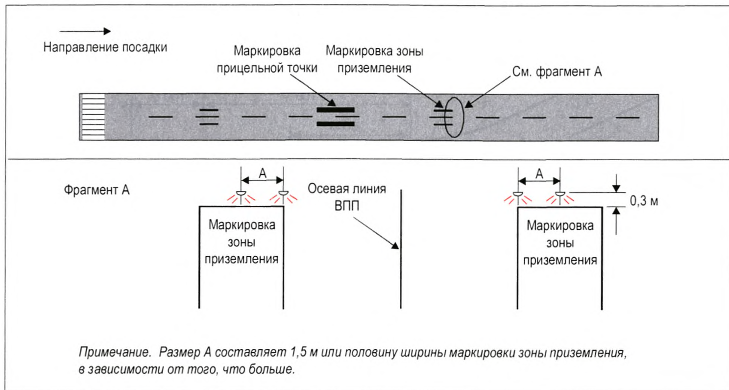
Рис. 5-24. Простые огни зоны приземления
