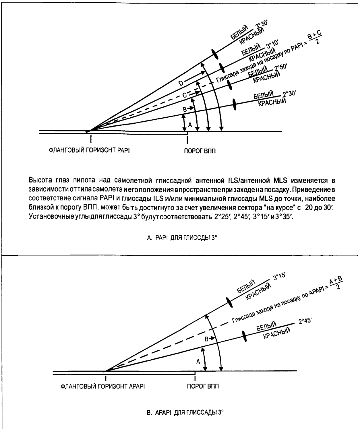
Рис. 5-20. Световые лучи и установка углов возвышения PAR и APAR
