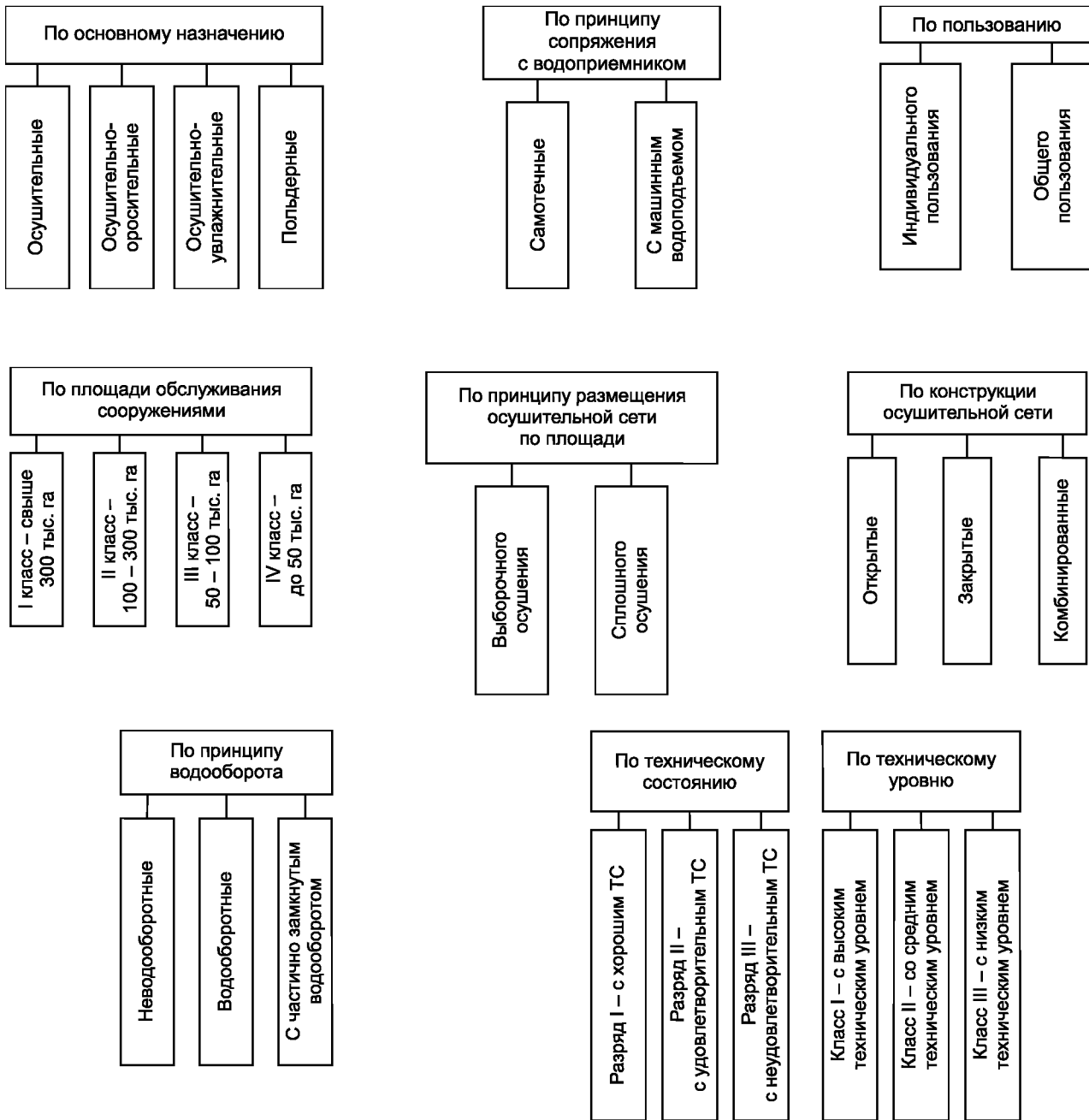
Рисунок Б.3 — Классификация осушительных систем
