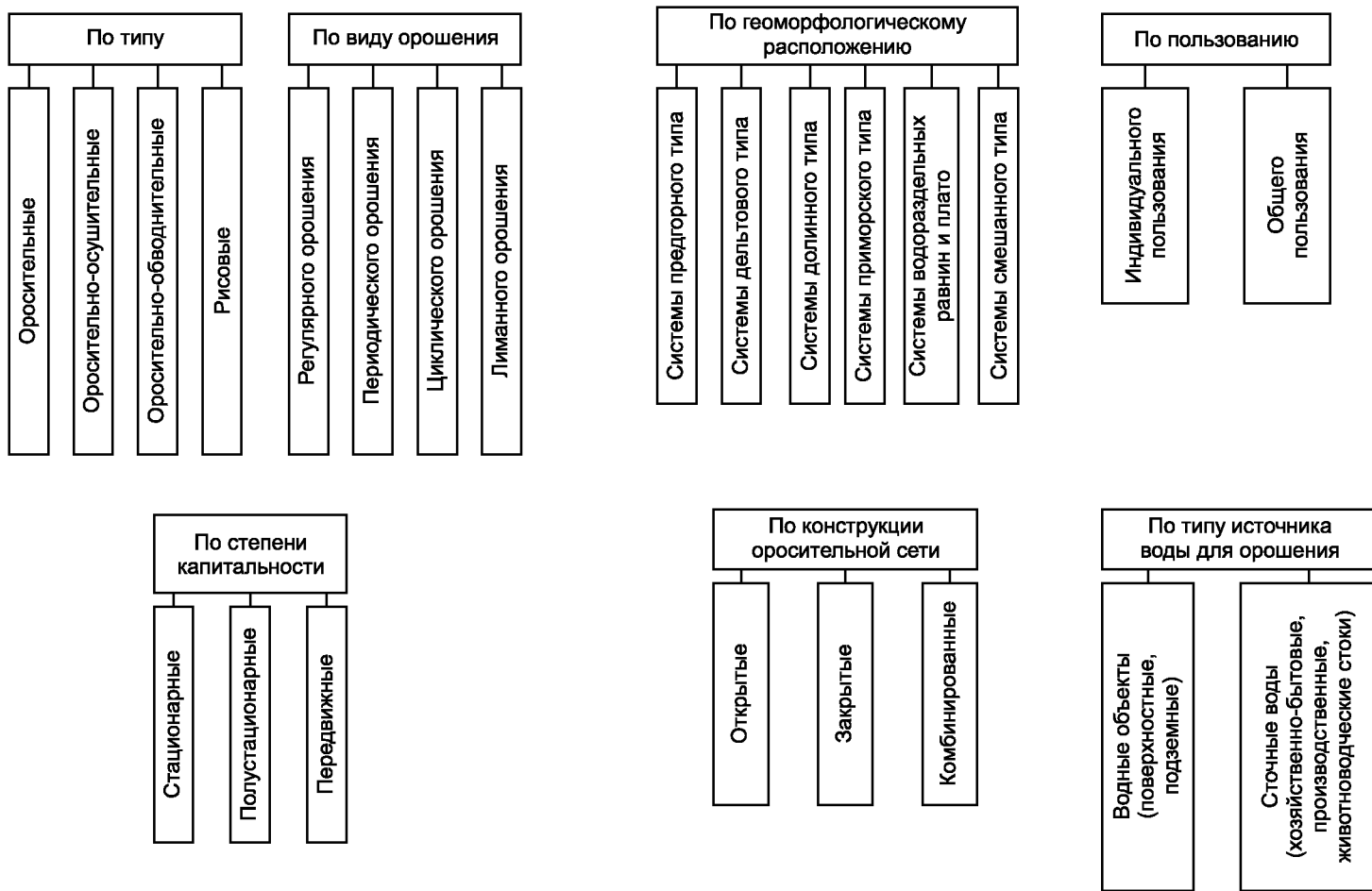
Рисунок А.3 — Классификация оросительных систем
