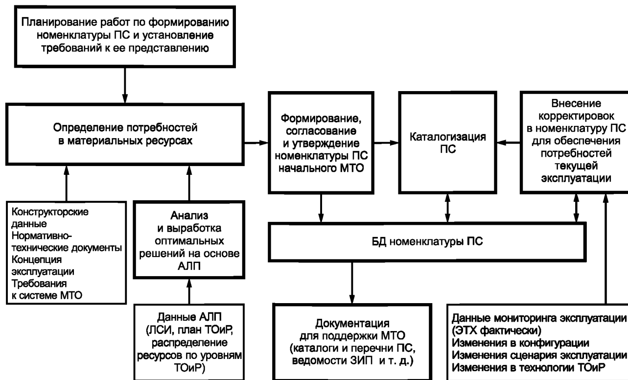
Рисунок А.1 — Типовая схема работ по формированию номенклатуры предметов снабжения
