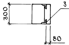
2-2 М 1:20
