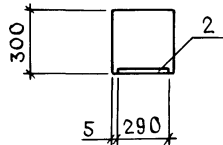
1-1 М 1:20
