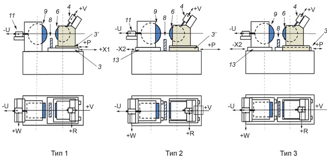
Рисунок 2 — Примеры конфигураций бесцентрового шлифовального станка
