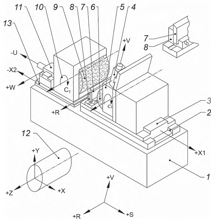
Рисунок 1 — Пример бесцентрового шлифовального станка
