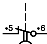
Размыкающий контакт с замедлением при замыкании
