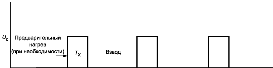
Профиль напряжения управления, U_c
