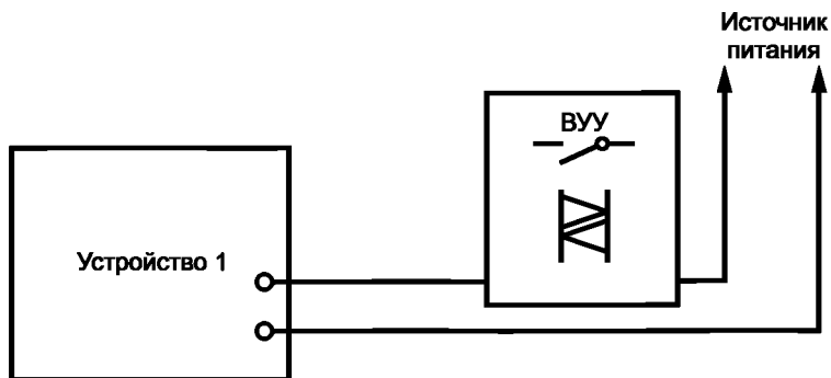
Рисунок G.3 — Раздельные вводы для источника питания и цепи управления
