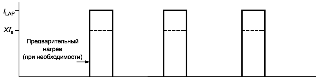
Профиль испытательного тока
