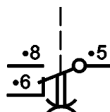
Переключающий контакт с замедлением в обоих направлениях
