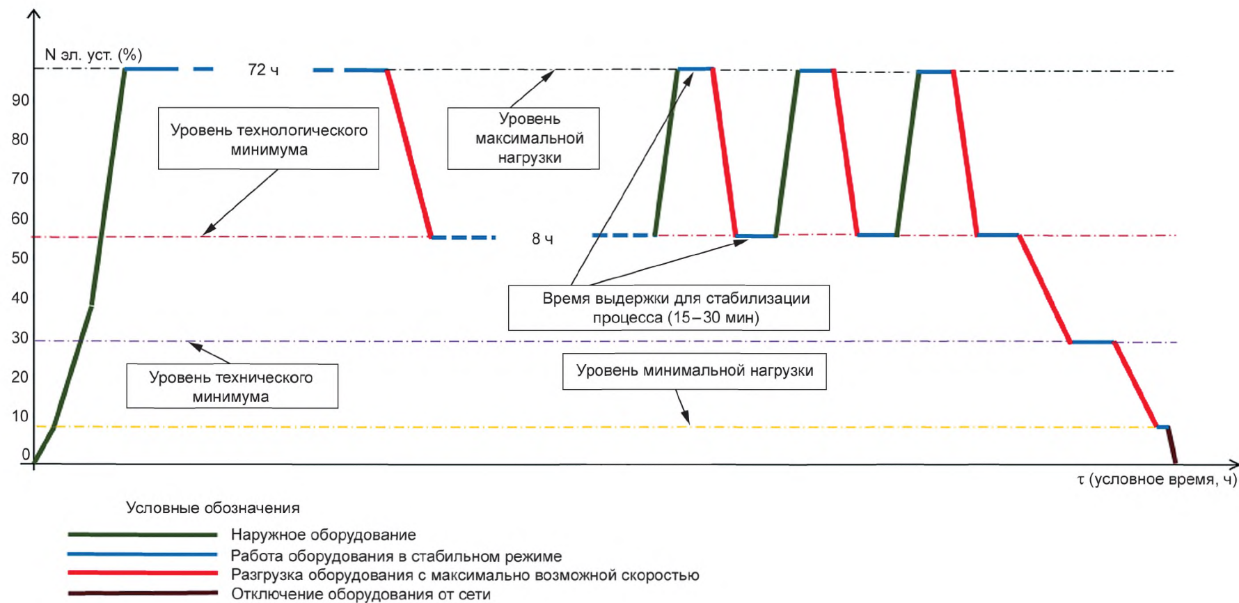
Рисунок Е.1 — Технологический график проведения комплексного опробования и иных этапов комплексных испытаний оборудования энергоблока по определению его общесистемных параметров и характеристик
