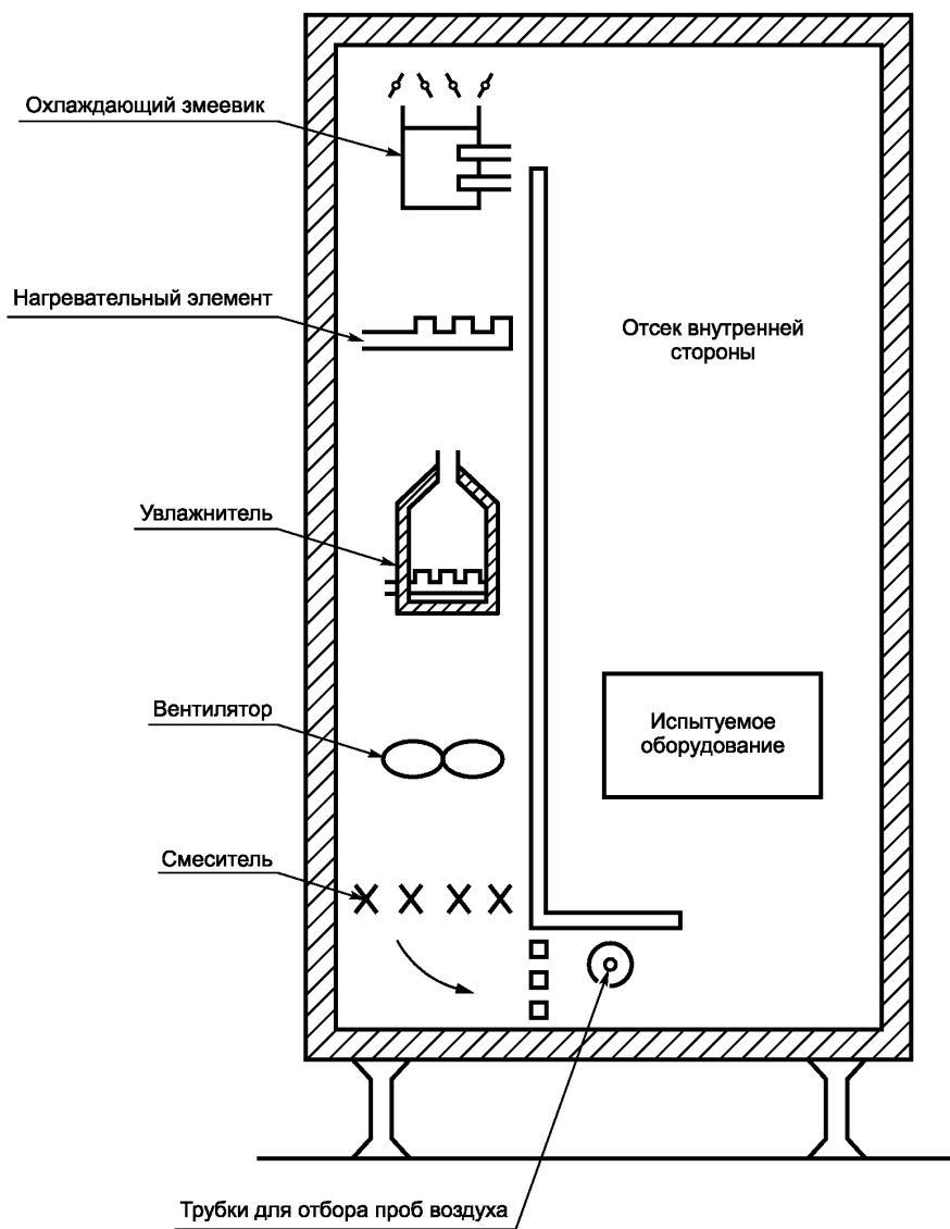
Рисунок Е.1 — Типичный калиброванный калориметр комнатного типа
