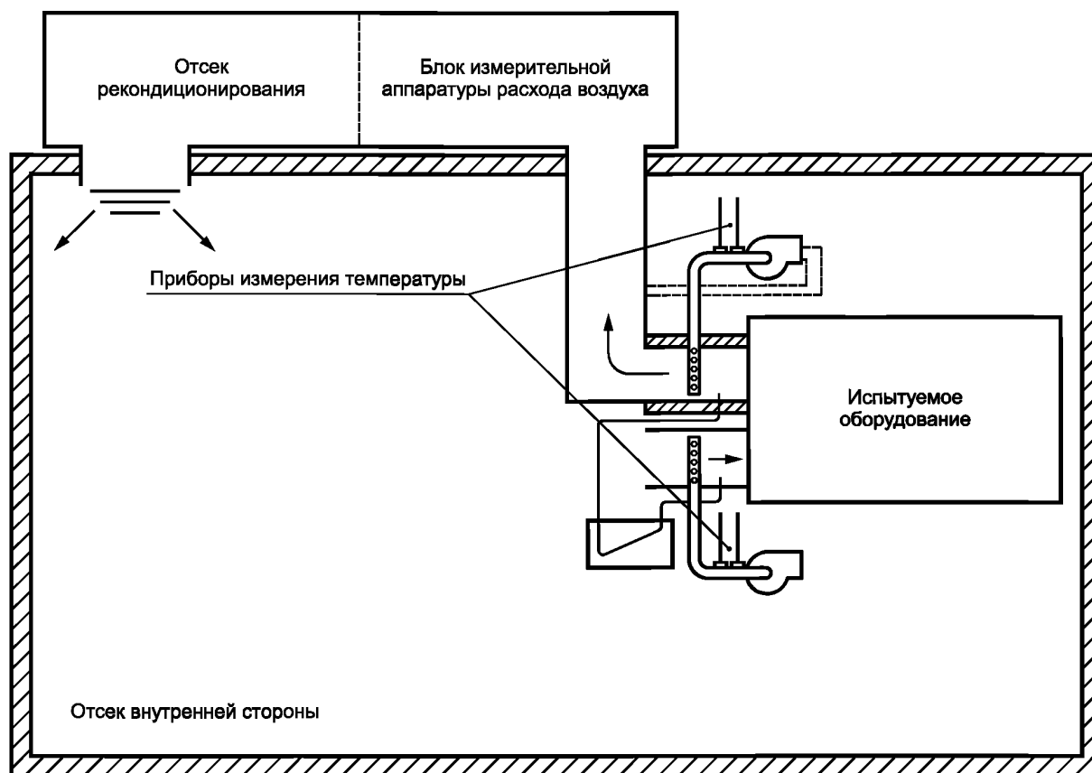
Рисунок F.4 — Компонка оборудования испытательной камеры для проведения испытаний методом комнаты
