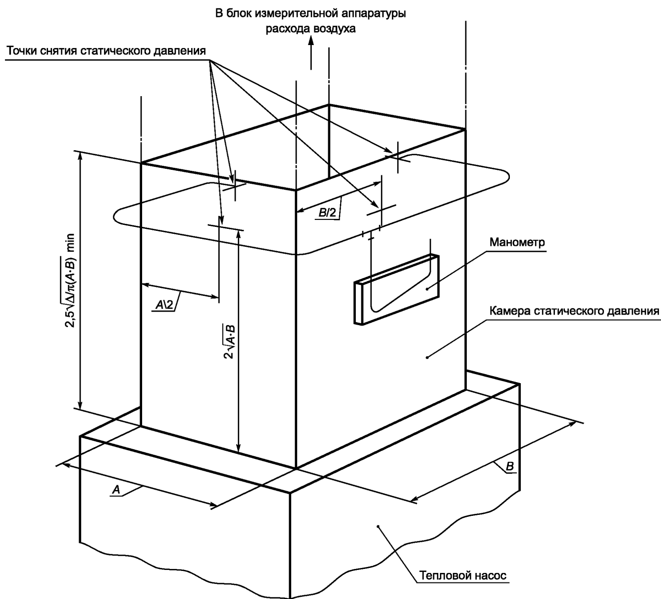
Рисунок F.7 — Измерение внешнего статического давления
