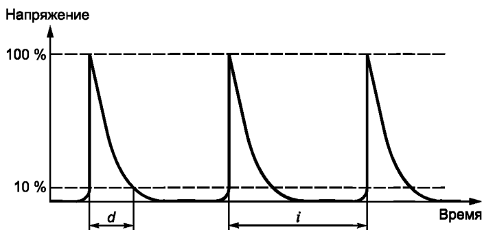
Рисунок 101 — Генерация импульсного искрового поджига
