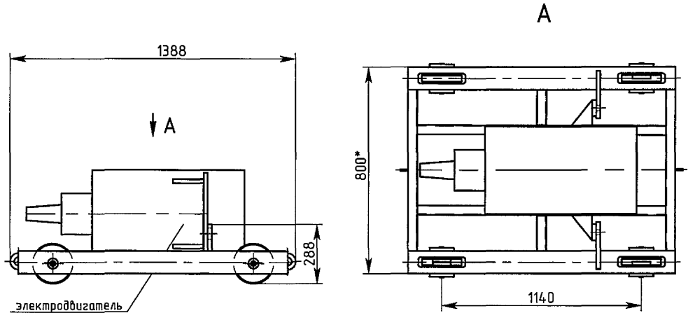
Масса тележки для выкатки электродвигателя - 242 кг
