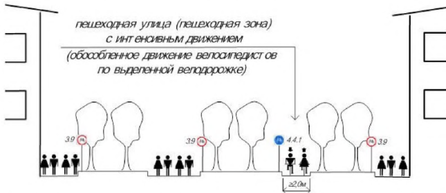
Рисунок 8.16 - Ограничение доступа велосипедистов в пешеходной зоне
