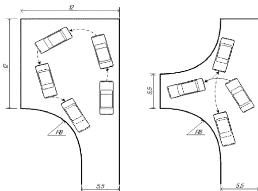
Рисунок 7.12 - Схема обустройства тупиков
