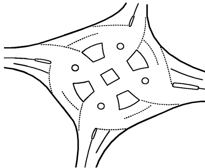
Рисунок 5.5 - Пересечение канализированного типа со сложной планировкой (Вариант №5)
