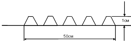
Рисунок 4.2 – Шумовые полосы из пластичных материалов
