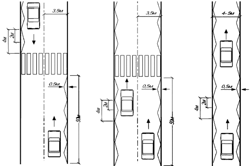
Рисунок 3.6 - Параметры зигзагообразной разметки
