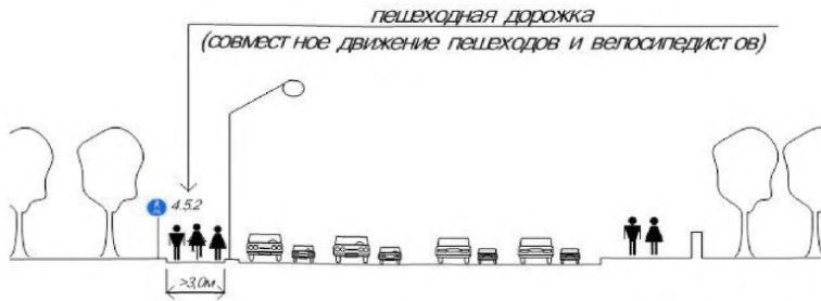
Рисунок 8.13 - Ограничение доступа велосипедистов к пешеходной дорожке
