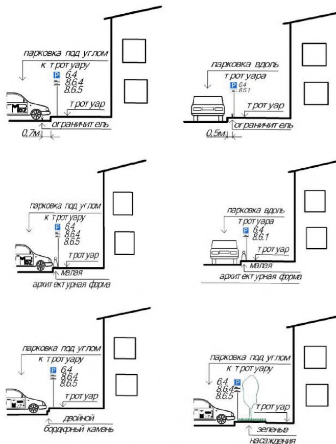
Рисунок 8.4 – Ограничение доступа автомобилей к тротуару при использовании ограничителей, малых архитектурных форм, зеленых насаждений при различных
