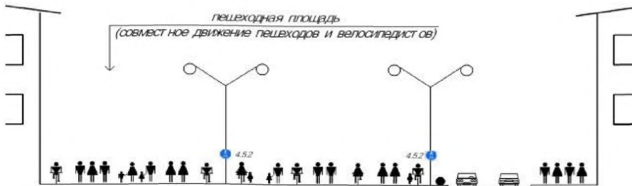
Рисунок 8.14 - Ограничение доступа велосипедистов к территории пешеходной площади
