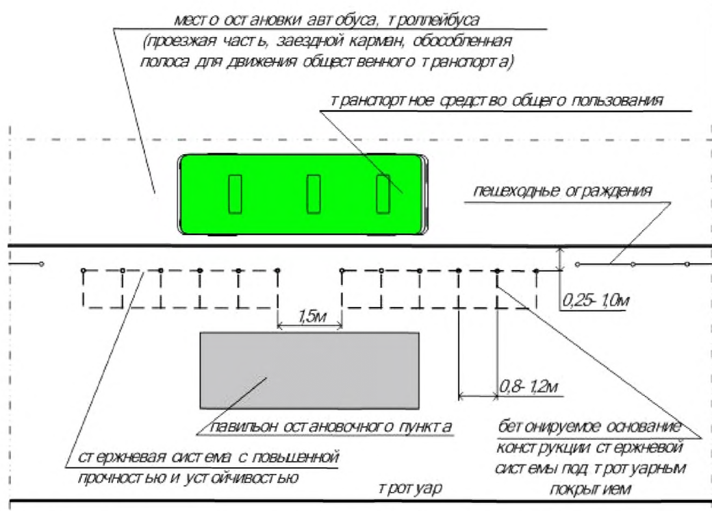
Рисунок 8.3 - Ограничение доступа автомобилей к территории остановочного комплекса
