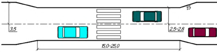
Рисунок 2.4 – Симметричное сужение проезжей части с внешней стороны УДС (метод № 1)
