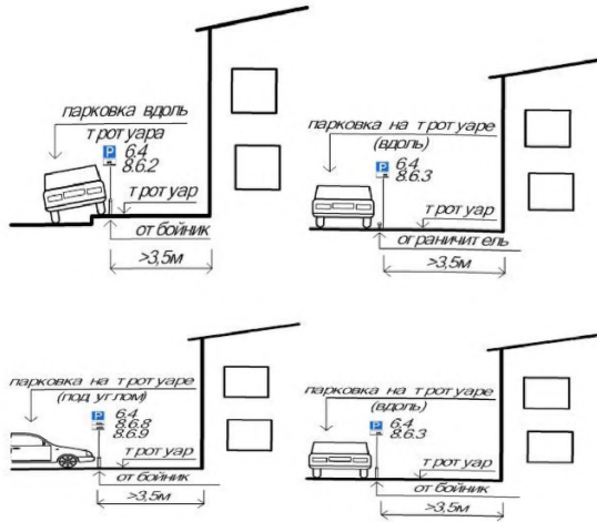
Рисунок 8.10 - Ограничение доступа автомобилей к тротуару
