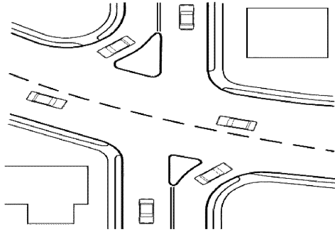
Рисунок 7.10 - Вариант обустройства для исключения сквозных проездов (пример № 3)
