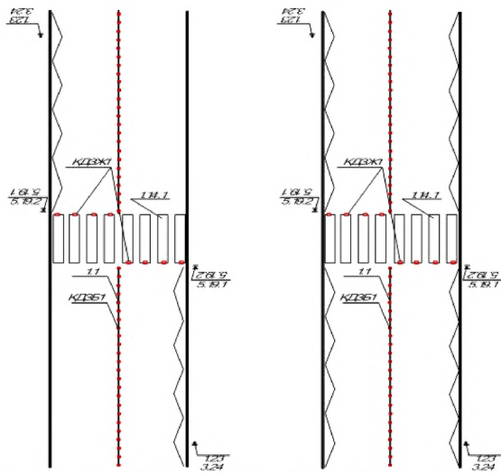
Рисунок 3.7 - Схема обустройства участков с зигзагообразной разметкой
