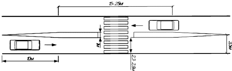
Рисунок 2.8 – Изменение эффективной ширины проезжей части (метод № 5)
