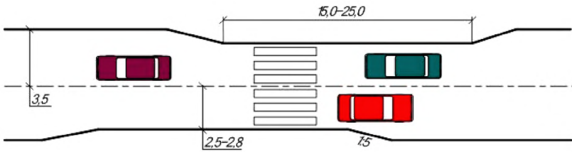
Рисунок 2.5 – Ассиметричное сужение проезжей части с внешней стороны УДС (метод № 2)
