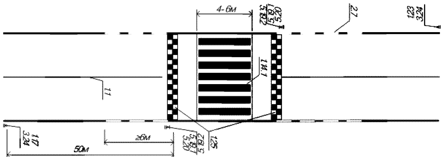
Рисунок 6.3 – Пример обустройства приподнятых пешеходных переходов
