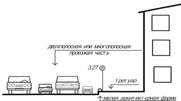
Рисунок 8.7 - Ограничение доступа автомобилей к тротуару с использованием малых архитектурных форм при наличии многополосной проезжей части дороги
