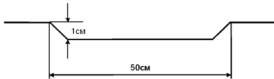
Рисунок 4.1 - Шумовые полосы, вырезанные на проезжей части
