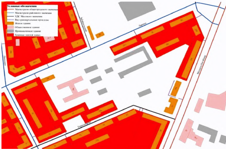
Рисунок 7.1 - Пример назначения границы жилой зоны
