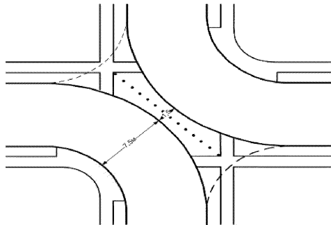
Рисунок 7.11 - Геометрические параметры диагональных перемычек
