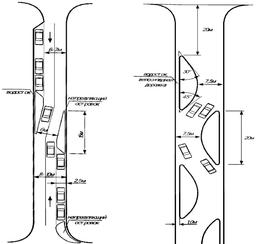
Рисунок 3.2 - Технические параметры организации зигзагообразного движения с трапециевидными и серповидными направляющими островками
