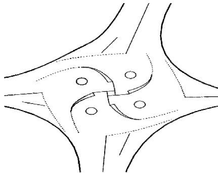
Рисунок 5.4 - Пересечение канализированного типа со сложной планировкой (Вариант №4)
