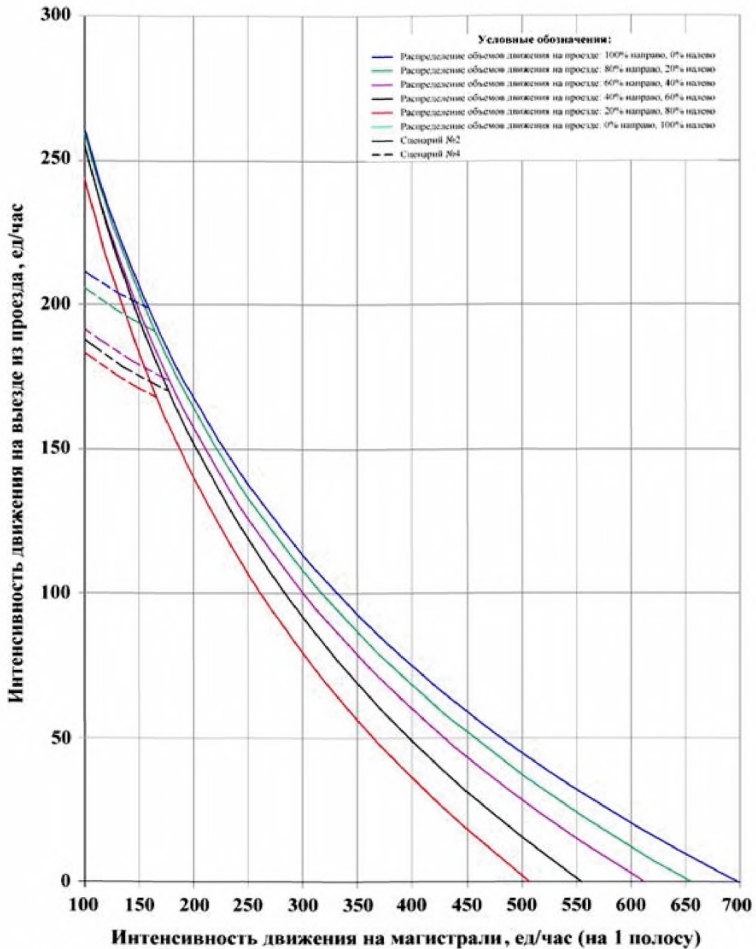
Рисунок 7.7 - Номограмма выбора максимального объема движения, проходящего на один проезд при совместном движении пешеходов и автомобилей по территории проездов-проходов
