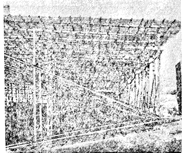
Рис. 22. Армирование блока нижними и верхними сетками с поддерживающими конструкциями между ними
