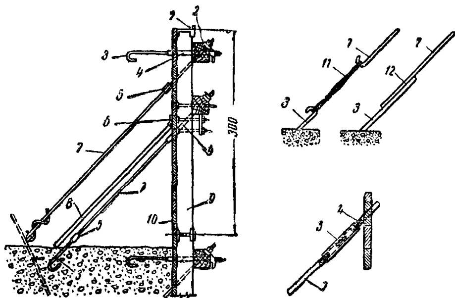
Рис. 14. Крепление опалубки наклонными тяжами с болтами на одном конце
