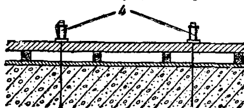
Рис. 13. Крепление опалубки горизонтальными тяжами со стаканами на одном конце 1 — натяжная гайка; 2 — сварка; 3 — стяжка; 4 — стакан
