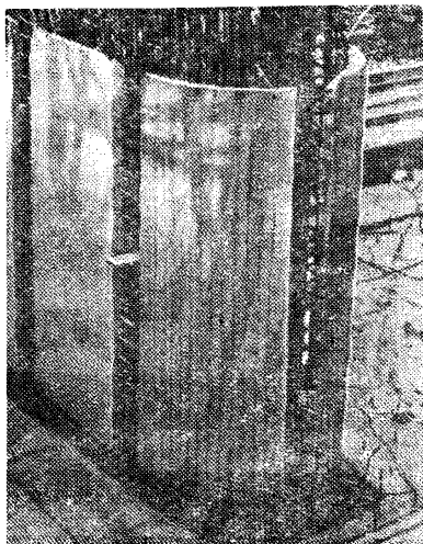
Рис. 20. Оголовок бычка верхнего бьефа. Армированные криволинейными сетками
