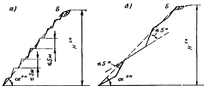
Рисунок Д.1 – Схемы поперечного профиля – тип I
