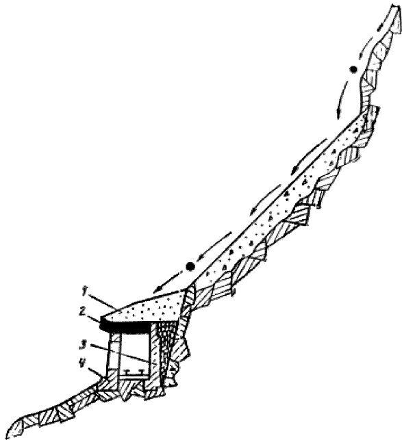
Рисунок 4 – Схема противообвальнoй галереи
