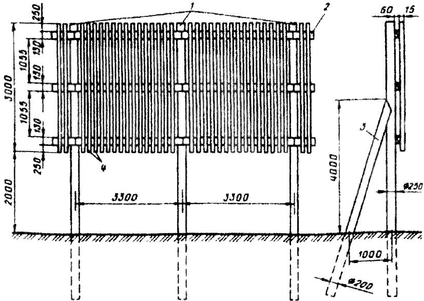
Рисунок А.6 – Схема снегопередувающего забора
