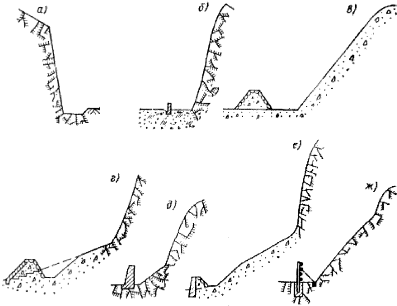
а) путевая траншея; б) улавливающая полка с бордюром; в) улавливающий вал у подошвы склона; г) улавливающий вал на склоне; д) оградительная улавливающая стена; е) улавливающая стена; ж) улавливающая сетка
