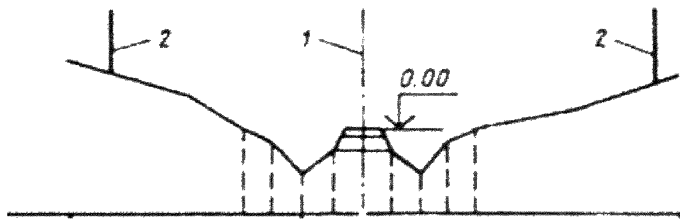
Рисунок Б.3 – Схема разбивки контрольного снегомерного створа
