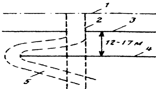
1 – ось пути; 2 – переезд; 3 – первый ряд щитовой линии; 4 – второй ряд щитовой линии; 5 – отведенная дорога
