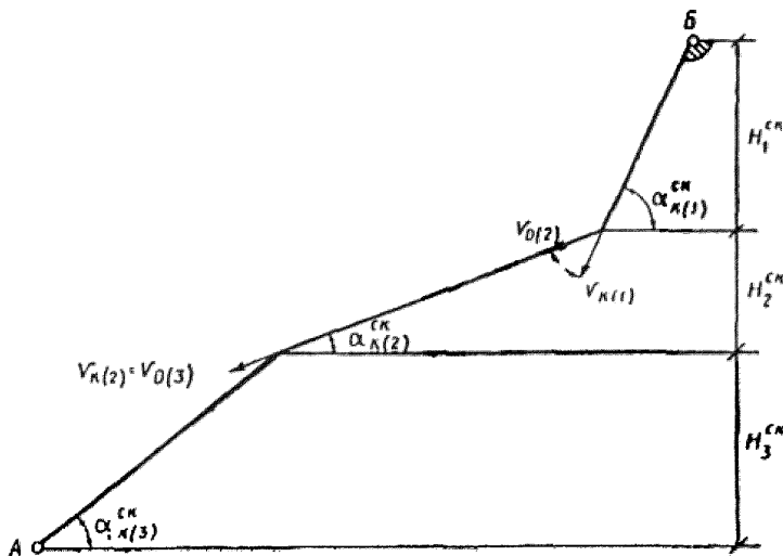
Рисунок Д.3 – Схема поперечного профиля – тип III
