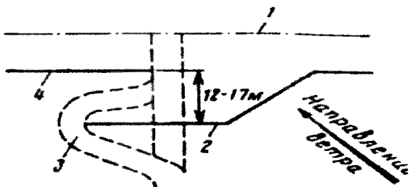
1 – ось пути; 2 – отведенная линия щитов; 3 – отведенная дорога; 4 – щитовая линия
