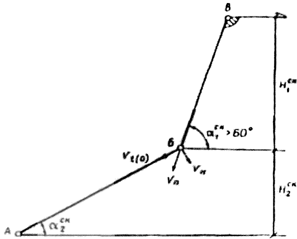
Рисунок Д.4 – Схема поперечного профиля – тип IV
