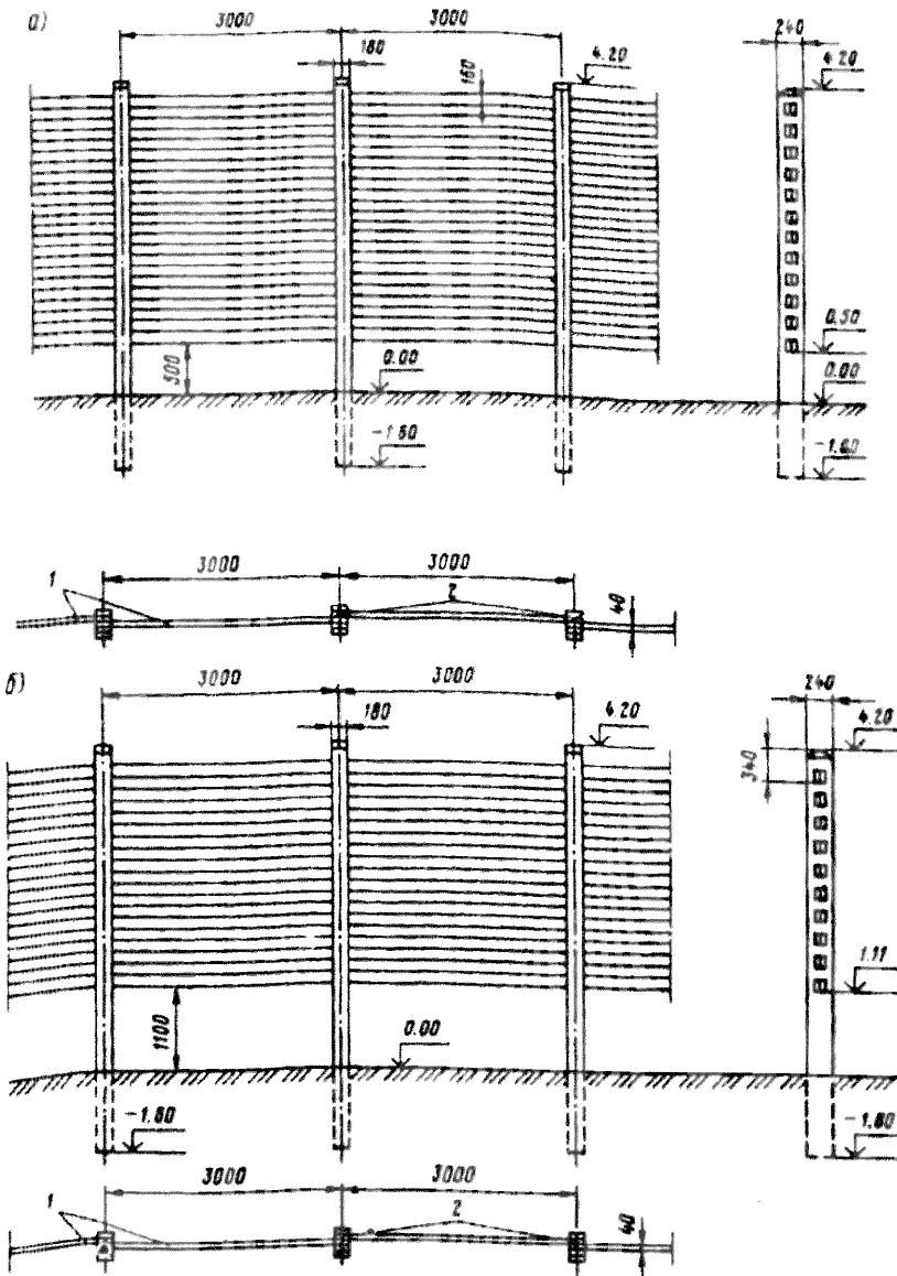
Рисунок А.4 Схемы путевого (а) и полевого (б) железобетонных снегозадерживающих заборов сборной конструкции
