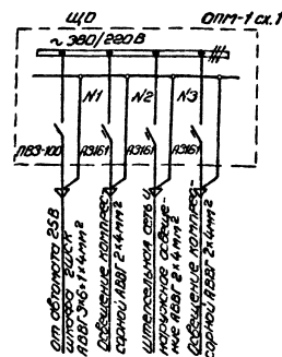
Щиток освещения
