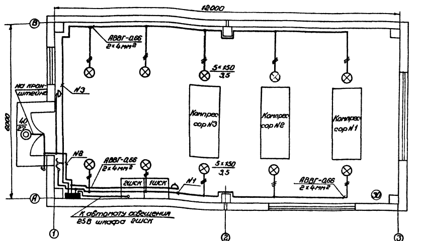
План сети освещения
