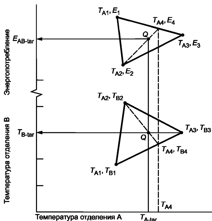
Рисунок Е.4 — Схематическое представление интерполяции посредством триангуляции
