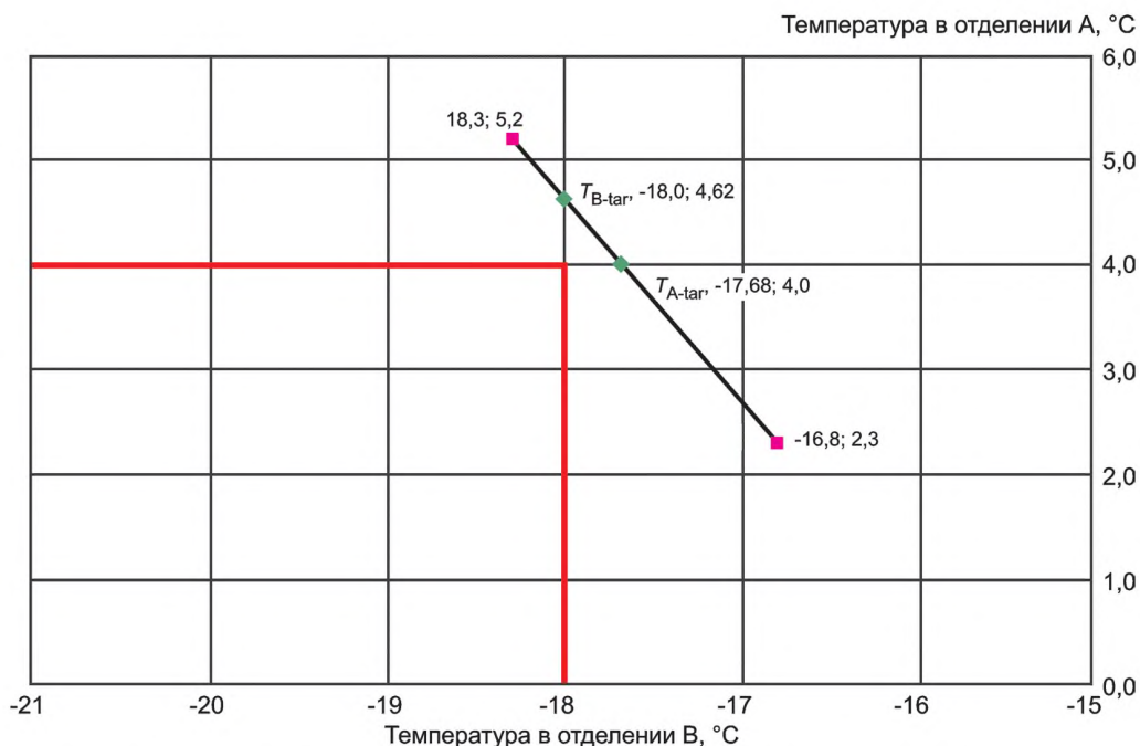
Рисунок I.5 — Пример интерполяции, когда ни в одной из точек испытаний оба отделения не имеют температуру ниже целевой температуры (нет допустимых результатов)
