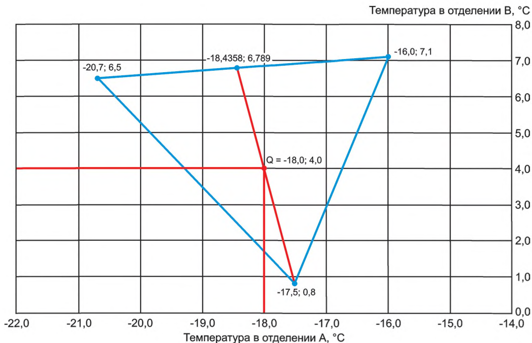
Рисунок 1.8 — Пример триангуляции (температуры)
