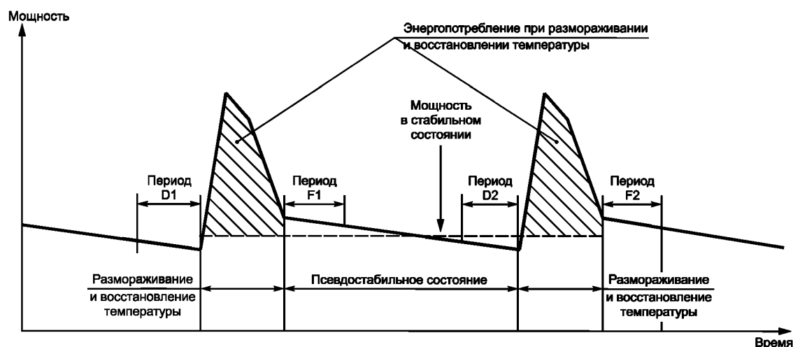
Рисунок К.1 — Особый случай SS2 — когда работа в стабильном состоянии не достигается между периодами размораживания и восстановления температуры и стабильность по приложению С не может быть установлена
