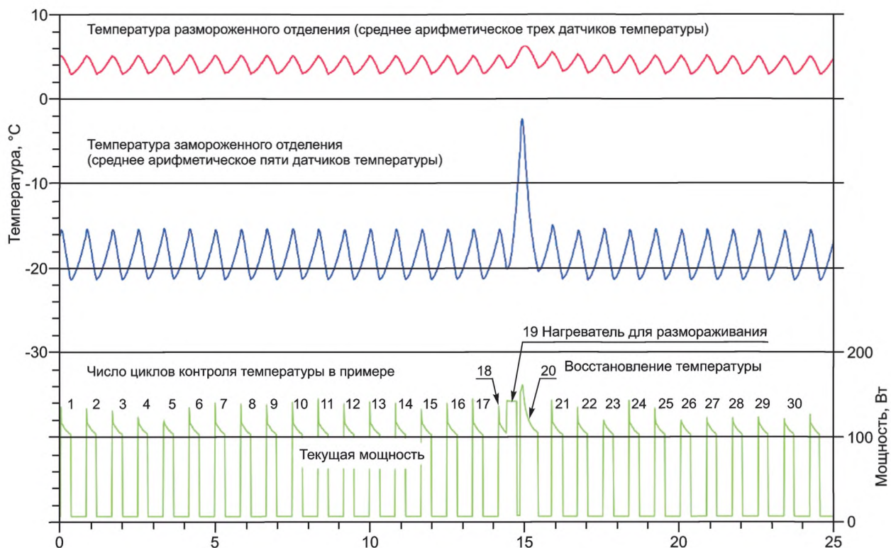
Рисунок I.10 — Пример данных по мощности и температуре
