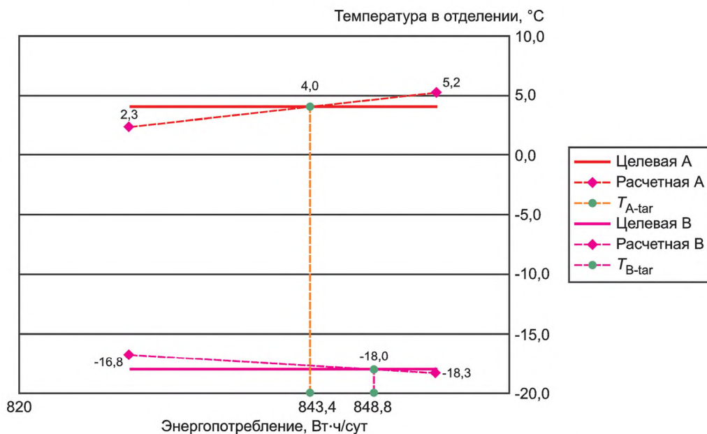
Рисунок I.6 — Пример интерполяции, когда ни в одной из точек испытаний оба отделения не имеют температуру ниже целевой температуры (нет допустимых результатов)
