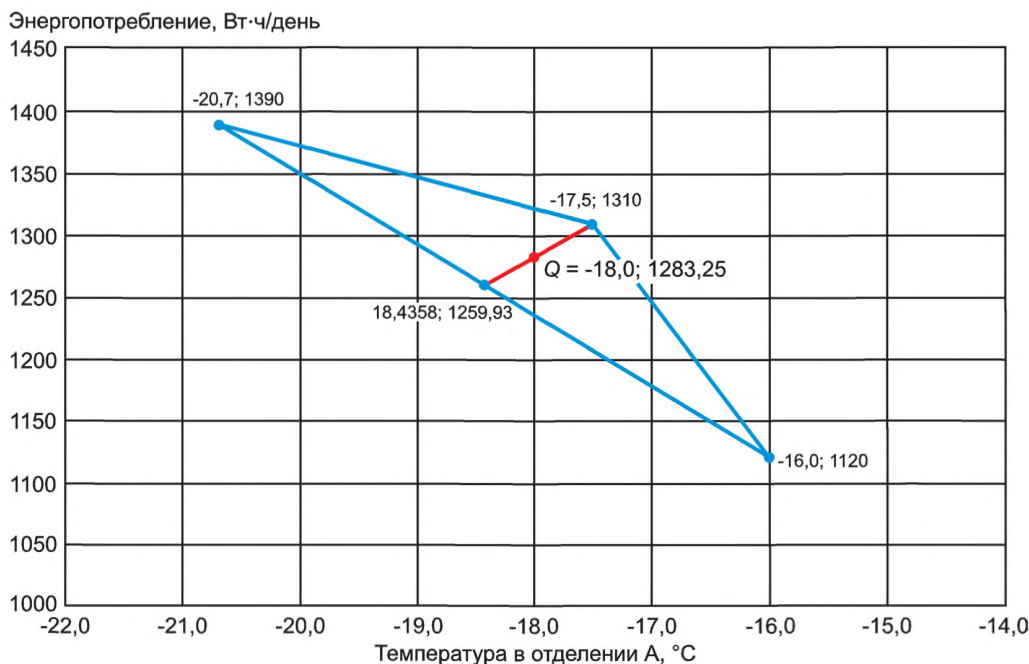
Рисунок 1.9 — Пример триангуляции (температура и энергопотребление)
