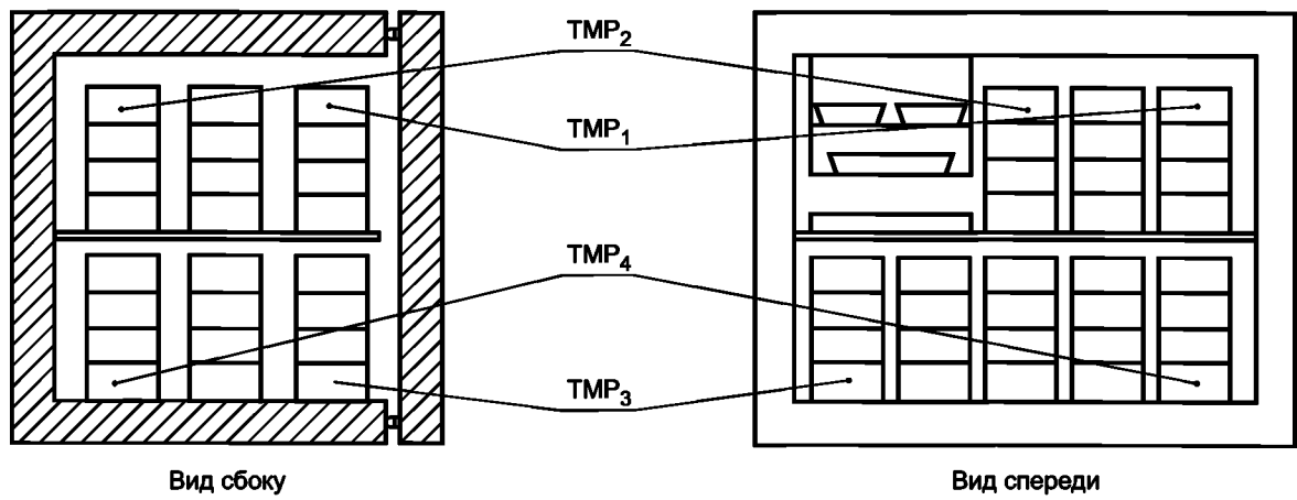
д) Определение полной ширины с закрепленными подставками для форм для льда бункерами для льда с зеркальными расположениями М-пакетов
