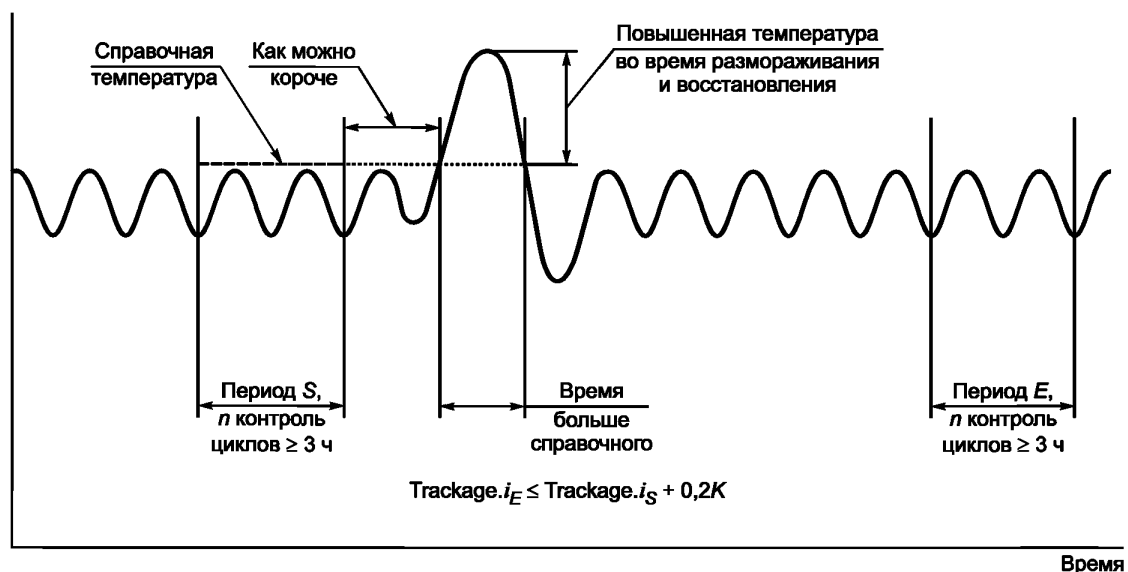
Рисунок 3 — Последовательность испытаний хранения
