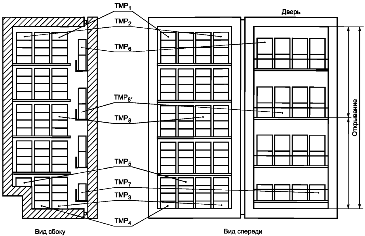
е) Высокое отделение, показывающее добавление среднего М-пакета
