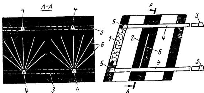
Рис. 3.35. Схема дегазации мощного крутого пласта скважинами, пробуренными по пласту из промежуточных квершлагов:
