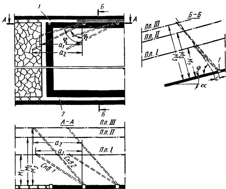
Рис. 3.4. Схема дегазации подрабатываемых угольных пластов при столбовой системе разработки (обратный порядок отработки): 1 — вентиляционный штрек дегазируемой лавы; 2 — откаточный штрек дегазируемой лавы
