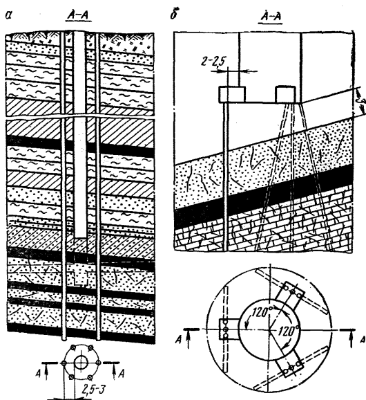
Рис 2.1. Схема дегазации газоносного массива при проходке вертикальных выработок: а — скважины бурятся с поверхности; б — скважины бурятся из специальных камер
