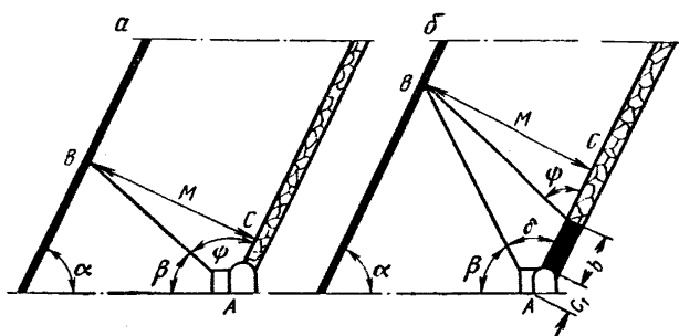
Рис. 3.27. Схема к определению направления скважины, пробуриваемой из откаточного штрека на вышележащий сближенный пласт: a — при отсутствии целика (бутовой полосы) над штреком; б — при наличии целика (бутовой полосы) над штреком
