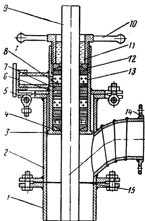
Рис. 7.1. Герметизатор
