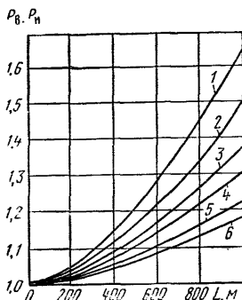
Рис. 4.8. Зависимость коэффициента подсосов воздуха P_B в трубопровод и утечек P_n от диаметра d , длины L и качества уплотнения трубопровода: 1 — k=0,0004 , d=0,5 м; 2 — k=0,0004 , d=0,6 м; 3 — k=0,0004 , d=0,7 м; 4 — k=0,0002 , d=0,5 м; 5 — k=0,0002 , d=0,6 м; 6 — k=0,0002 , d=0,7 м
