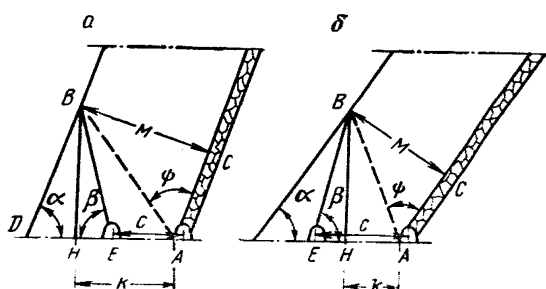
Рис. 3.28. Схема к определению направления скважины, пробуриваемой из группового откаточного штрека на вышележащий сближенный пласт, при отсутствии целика (бутовой полосы) над штреком: a — k > c ; б — k < c
