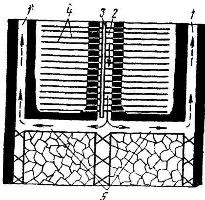
Рис. 2.15. Схема дегазации разрабатываемого пласта параллельно-одиночными горизонтальными пластовыми скважинами при столбовой системе разработки (вариант спаренные лавы по восстанию или падению):
