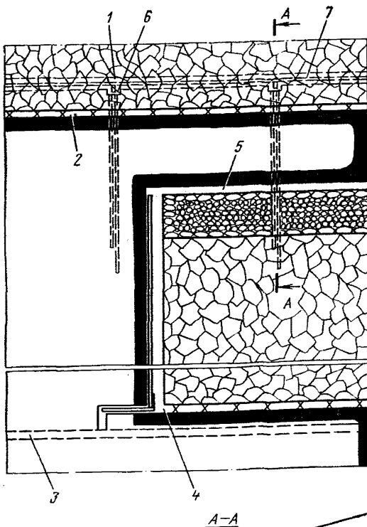
Рис. 36. Схема дегазации подрабатываемых угольных пластов скважинами при бурении скважин из полевых штреков:
