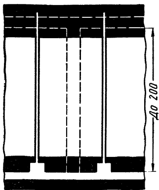
Рис. 2.4. Схема дегазации газоносного угольного массива барьерными скважинами при проведении коротких выработок по углю
