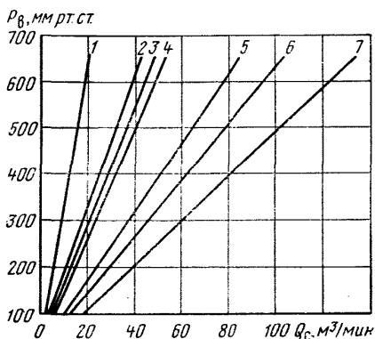
Рис. 7.8. Характеристики вакуум-насосов:
