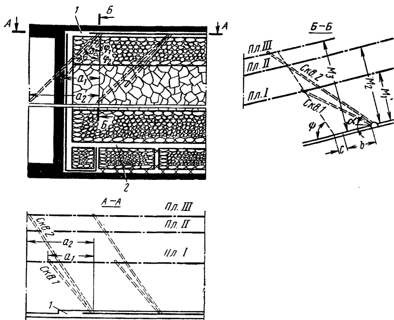
Рис. 3.2. Схема дегазации подрабатываемых угольных пластов скважинами, пробуренными с разворотом из вентиляционного штрека дегазуемой лавы, при сплошной системе разработки:
