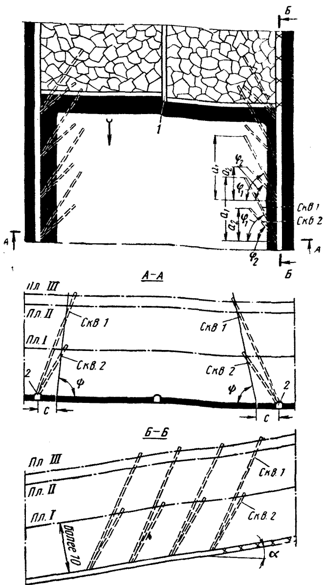
Рис. 3.5. Схема дегазации подрабатываемых угольных пластов при столбовой системе разработки с выемкой по падению или восстановлению пласта:
