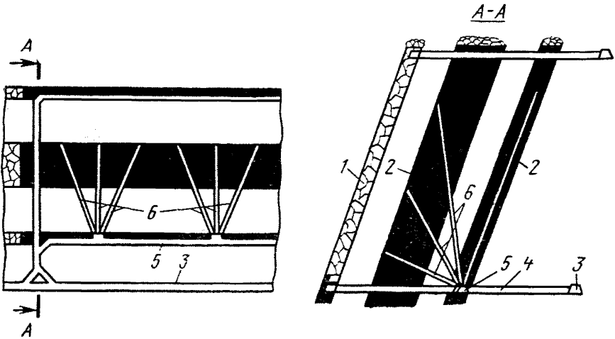
Рис. 2.20. Схема дегазации надрабатываемых крутых пластов веро-кустовыми скважинами, пробуренными из выработок одного из пластов свиты:
