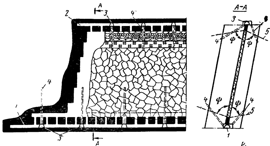
Рис. 3.22. Схема дегазации крутых близких пластов скважинами, пробуренными из выработок разрабатываемого пласта, при сплошной системе разработки:
