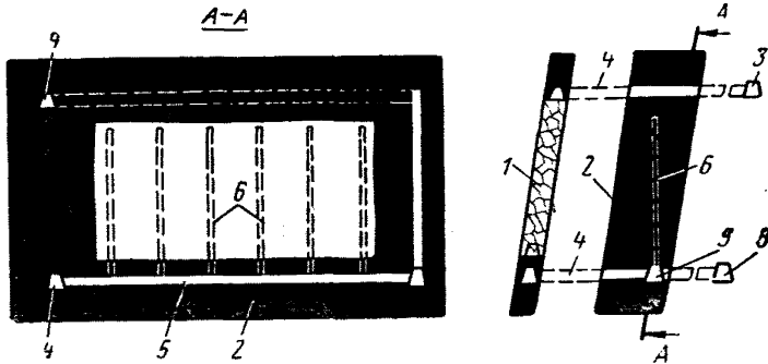
Рис. 3.34. Схема дегазации надрабатываемого мощного крутого пласта скважинами, пробуренными по надрабатываемому пласти из подготовительной выработки:
