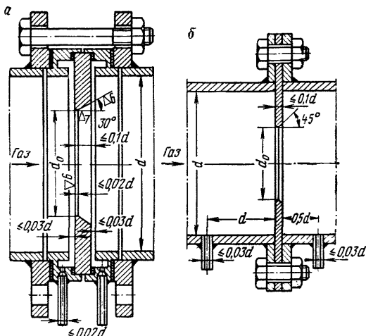
Рис. 7.10. Диафрагмы для замера расхода газа: а — нормальная; б — с замерами давлений на расстояниях d и 0,5 d от сужающего отверстия
