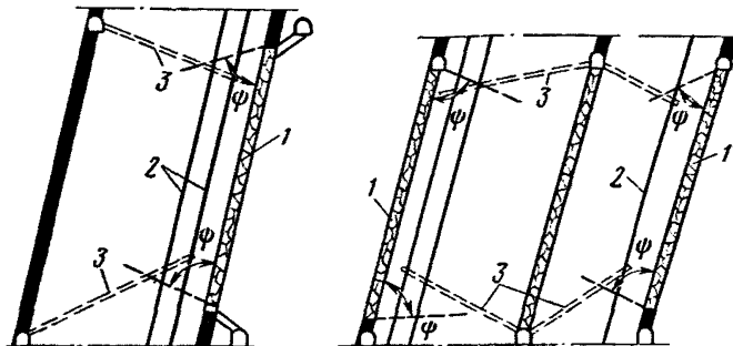
Рис. 3.24. Схема дегазации сближенных слоев скважинами, пробуренными из выработок пластов, соседних с разрабатываемым:
