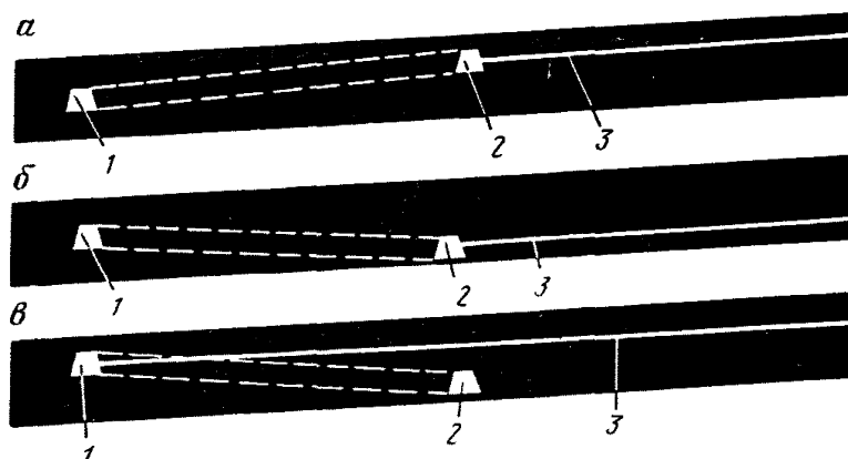
Рис. 2.22. Схема расположения дегазационных скважин при подготовке мощного пологого пласта с бурением скважин из: а — слоевого штрека верхнего слоя; б — слоевого штрека нижнего слоя; в — откаточного штрека; 1 — откаточный штрек; 2 — слоевые конвейерные штреки; 3 — дегазационные скважины
