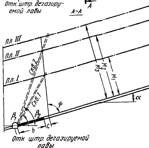
Рис. 3.1. Схема дегазации подрабатываемых угольных пластов скважинами, пробуренными без разворота из откаточного штрека дегазируемой лавы при сплошной системе разработки
