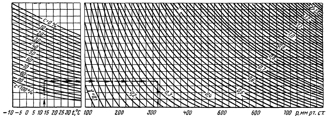
Рис. 7.9. Номограмма для определения объемной массы капируемого газа в зависимости от содержания в нем метана
