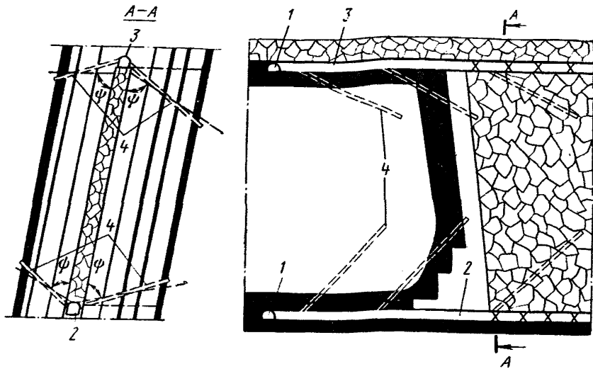
Рис. 3.23. Схема дегазации кривых сближенных слоев скважинами, пробуренными из выработок разрабатываемого пласта, при столбовой системе разработки:
