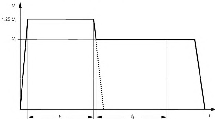
Рисунок 104 — Диаграмма зависимости испытательного напряжения от времени
