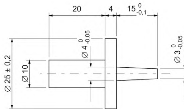
Рисунок 2 – Испытательный стержень
