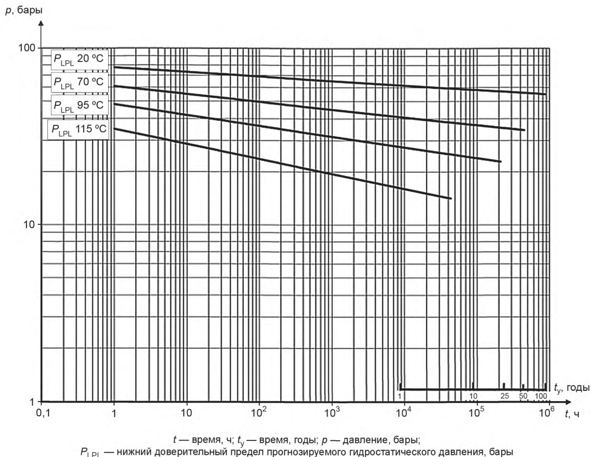
Рисунок А.1 — Пример графического представления длительной прочности армированной полимерной трубы
